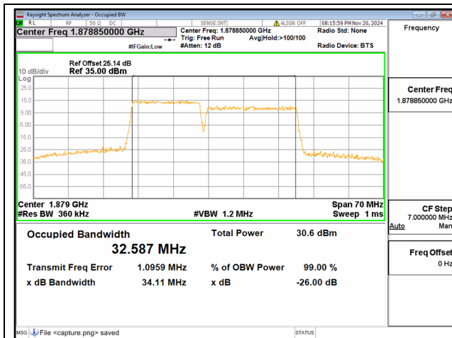
2C / 15+20MHz / QPSK/ Mid CH
