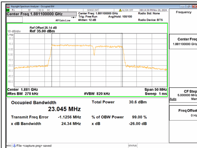
2C / 15+10MHz / QPSK/ Mid CH
