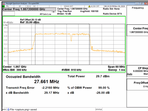
2C / 20+10MHz / 16QAM/ Low CH
