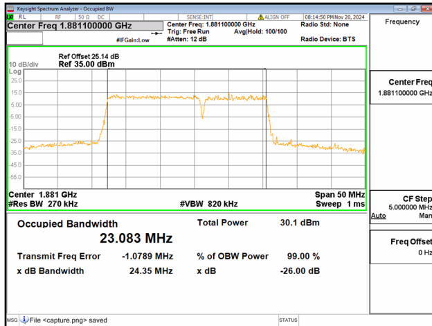
2C / 15+10MHz / 64QAM/ Mid CH
