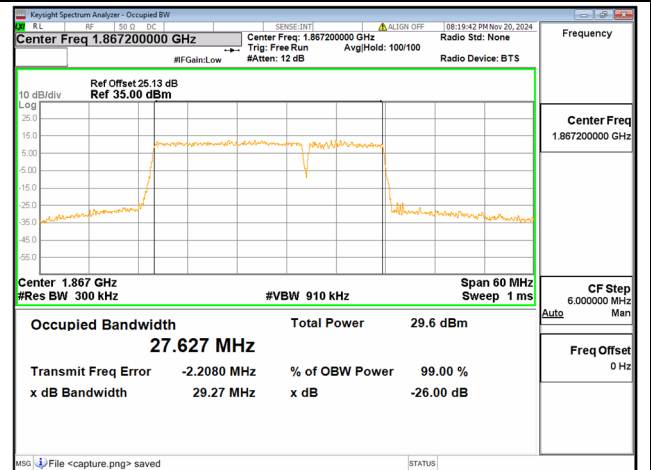
2C / 20+10MHz / 64QAM/ Low CH
