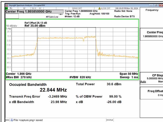
2C / 20+5MHz / QPSK/ Low CH
