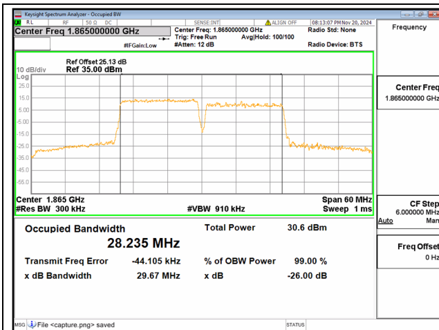
2C / 15+15MHz / QPSK/ Low CH
