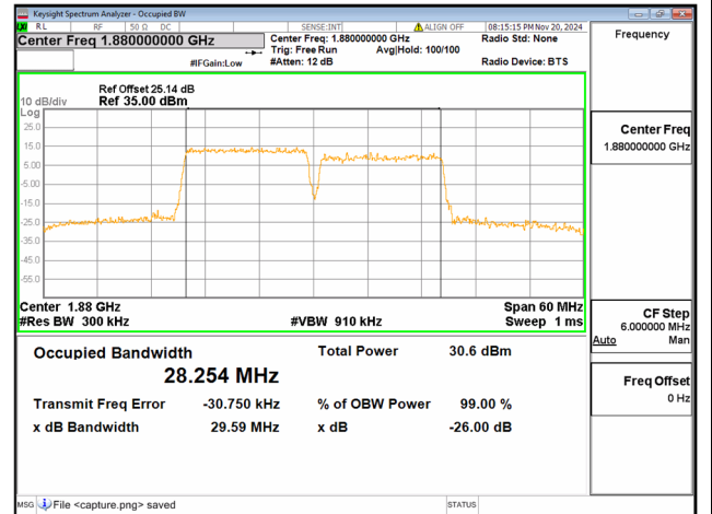
2C / 15+15MHz / QPSK/ Mid CH
