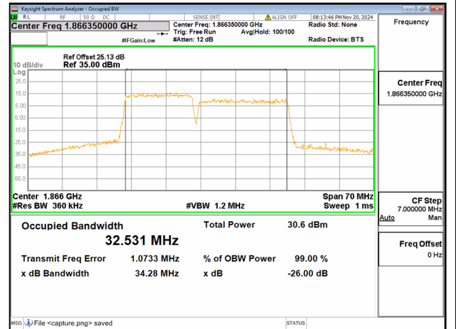
2C / 15+20MHz / QPSK/ Low CH
