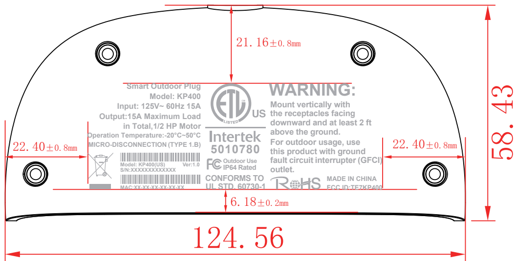
尺寸图
