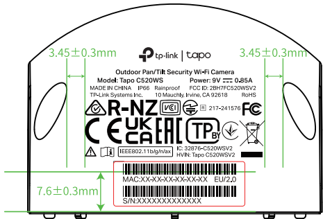
尺寸图
