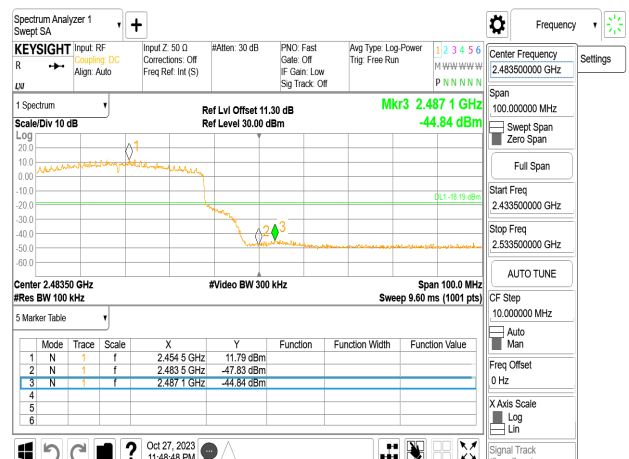
802.11be_40MHz_Chain0_2452MHz
