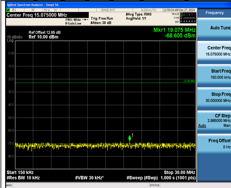
Band26 10MHz QPSK 26915 50RB#0 0.15~30 0.15~30
