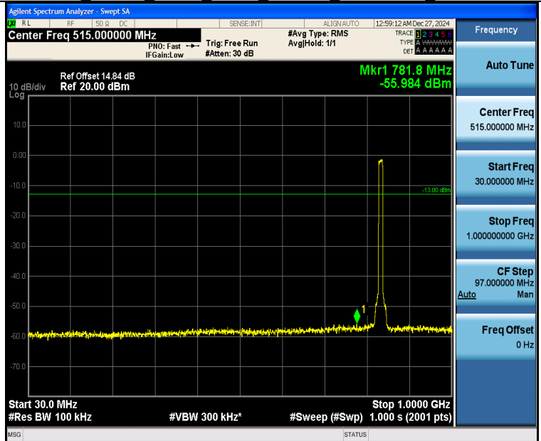
Band26 10MHz QPSK 26915 50RB#0 30~1000 30~1000
