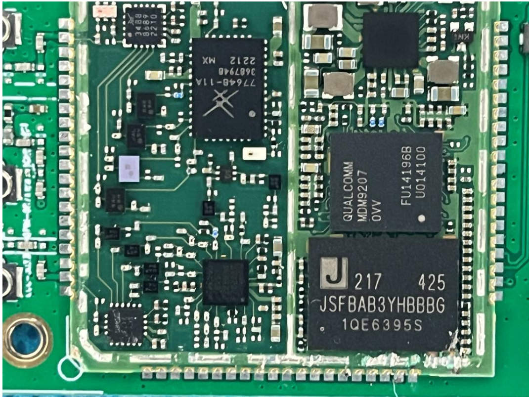
GSM/WCDMA/LTE Chip
