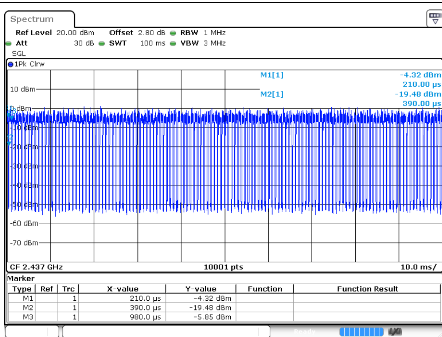
Test_Graph_802.11n40_ANT1_2437
