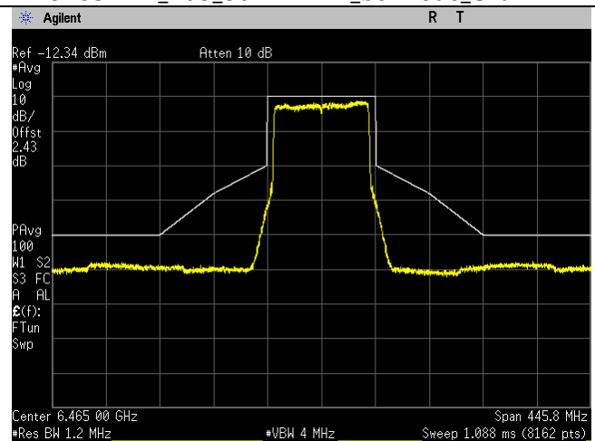
6465MHz_103_80MHz BW_be-mode_Chain 3
