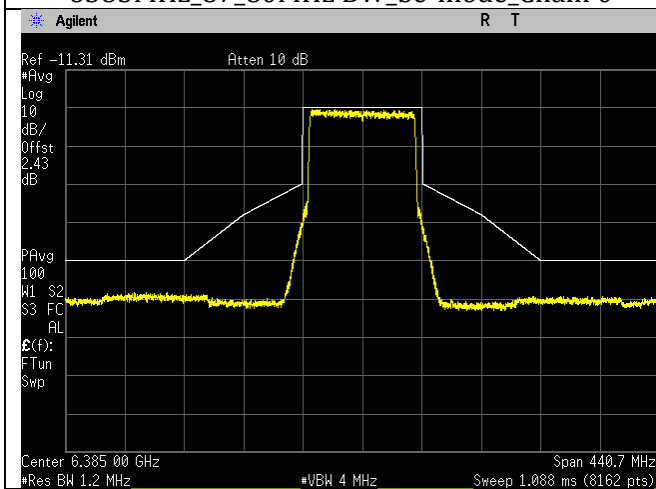
6385MHz_87_80MHz BW_be-mode_Chain 2
