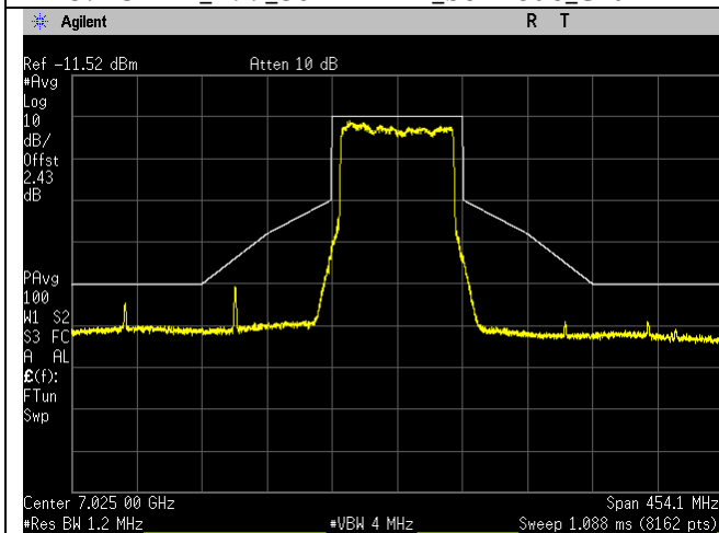
7025MHz_215_80MHz BW_be-mode_Chain 0
