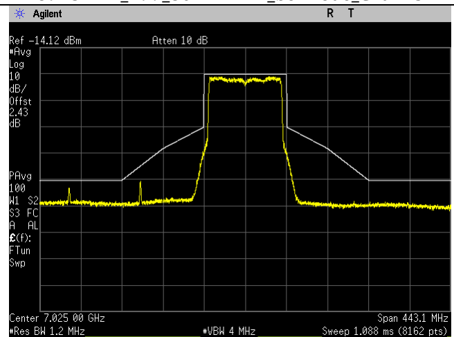
7025MHz_215_80MHz BW_be-mode_Chain 1
