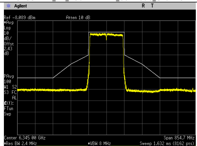
6345MHz_79_160MHz BW_be-mode_Chain 1
