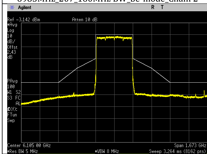
6105MHz_31_320MHz BW_be-mode_Chain 0
