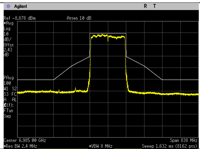
6985MHz_207_160MHz BW_be-mode_Chain 1
