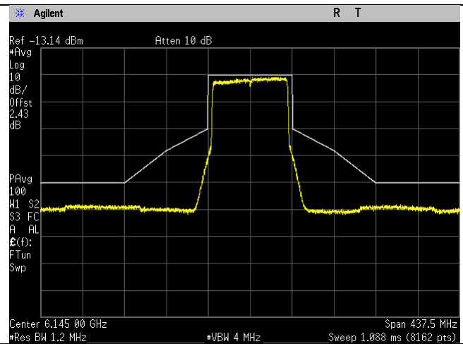
6145MHz_39_80MHz BW_be-mode_Chain 3
