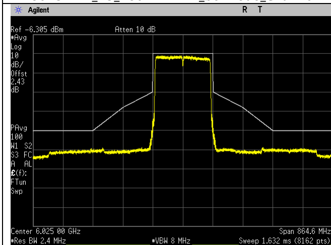
6025MHz_15_160MHz BW_be-mode_Chain 2
