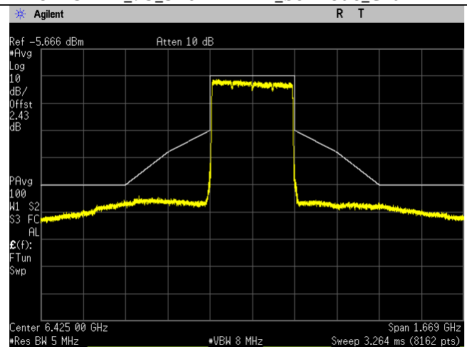
6425MHz_95_320MHz BW_be-mode_Chain 3
