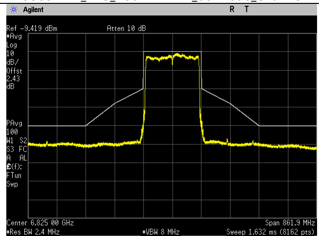
6825MHz_175_160MHz BW_be-mode_Chain 1
