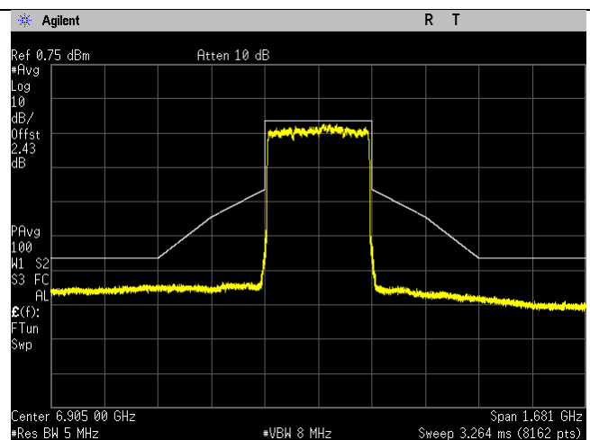
6905MHz_191_320MHz BW_be-mode_Chain 1
