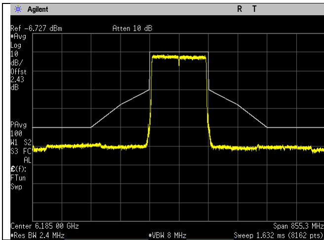
6185MHz_47_160MHz BW_be-mode_Chain 2
