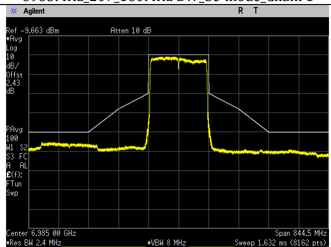
6985MHz_207_160MHz BW_be-mode_Chain 3
