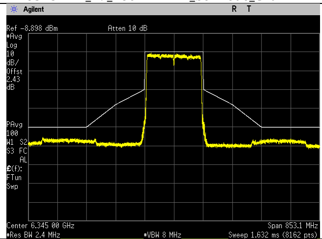
6345MHz_79_160MHz BW_be-mode_Chain 3
