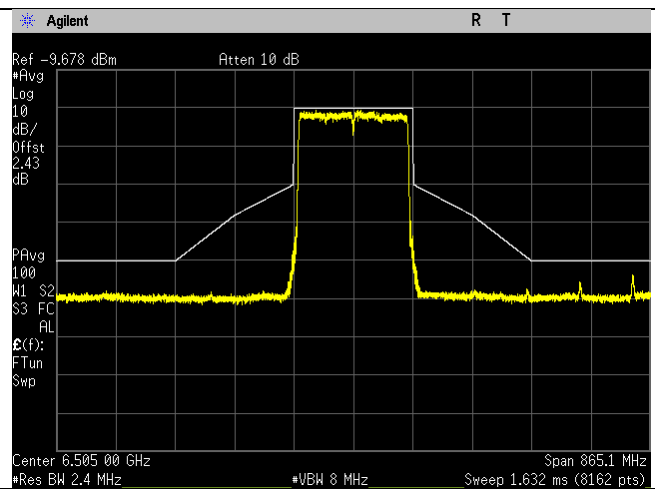
6505MHz_111_160MHz BW_be-mode_Chain 1
