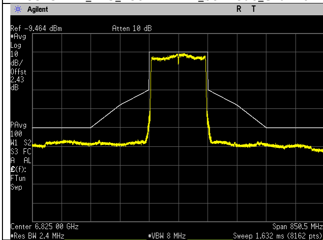
6825MHz_175_160MHz BW_be-mode_Chain 2
