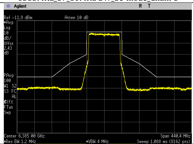
6385MHz_87_80MHz BW_be-mode_Chain 3
