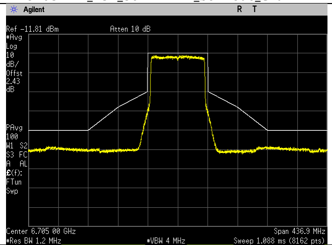
6705MHz_151_80MHz BW_be-mode_Chain 3
