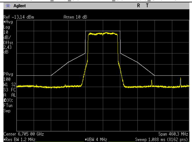
6705MHz_151_80MHz BW_be-mode_Chain 1
