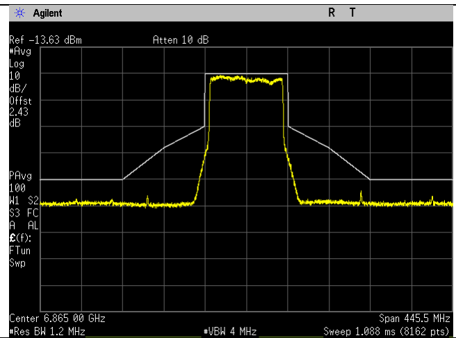
6865MHz_183_80MHz BW_be-mode_Chain 1
