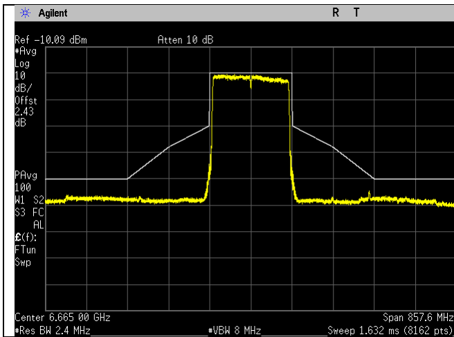
6665MHz_143_160MHz BW_be-mode_Chain 2
