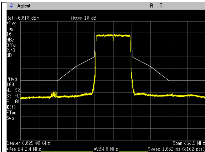
6025MHz_15_160MHz BW_be-mode_Chain 0
