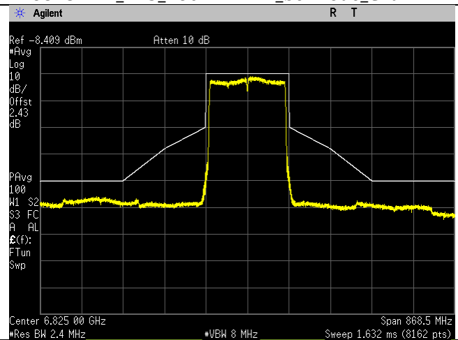
6825MHz_175_160MHz BW_be-mode_Chain 3
