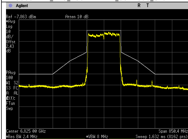
6825MHz_175_160MHz BW_be-mode_Chain 0
