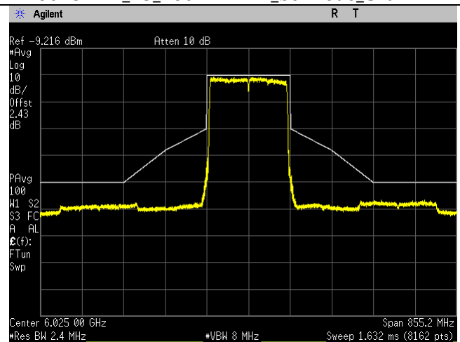
6025MHz_15_160MHz BW_be-mode_Chain 3
