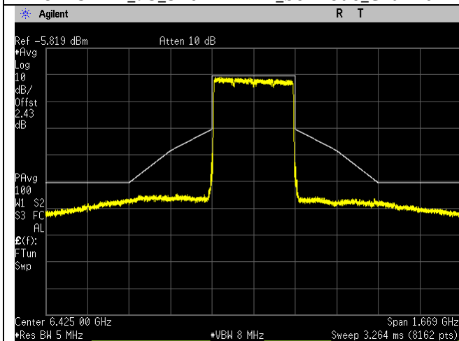
6425MHz_95_320MHz BW_be-mode_Chain 2
