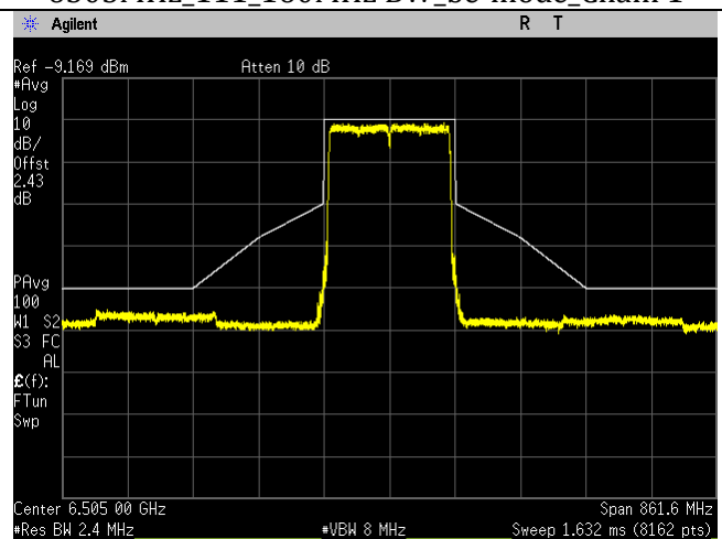
6505MHz_111_160MHz BW_be-mode_Chain 3
