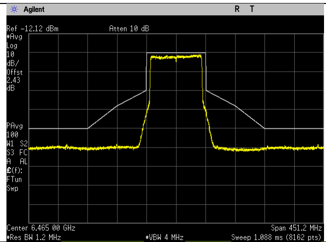
6465MHz_103_80MHz BW_be-mode_Chain 1
