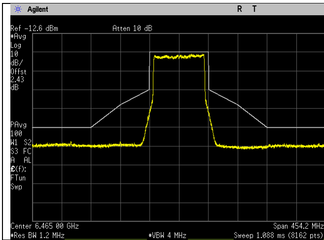
6465MHz_103_80MHz BW_be-mode_Chain 0
