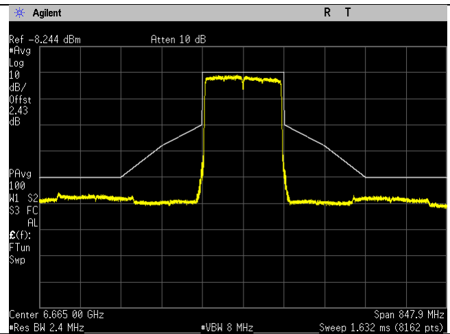
6665MHz_143_160MHz BW_be-mode_Chain 3
