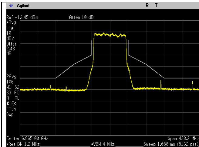
6865MHz_183_80MHz BW_be-mode_Chain 0
