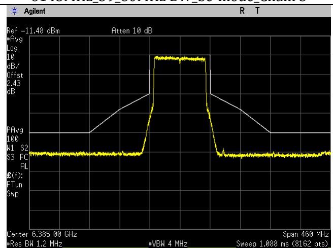
6385MHz_87_80MHz BW_be-mode_Chain 1
