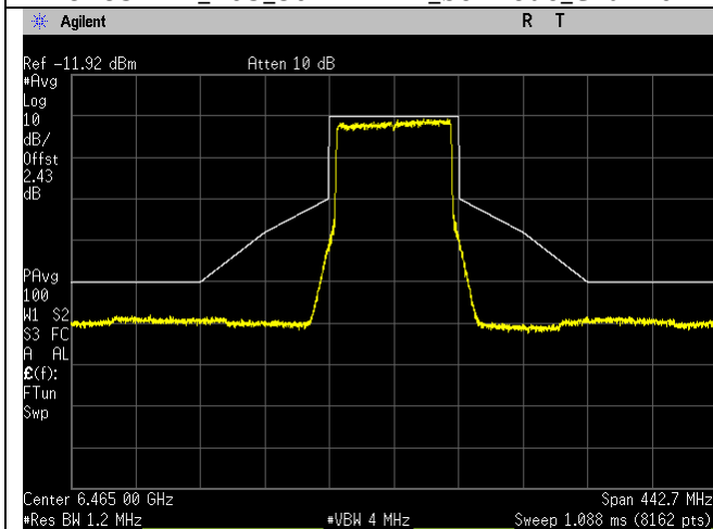
6465MHz_103_80MHz BW_be-mode_Chain 2
