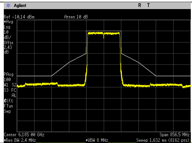
6185MHz_47_160MHz BW_be-mode_Chain 3
