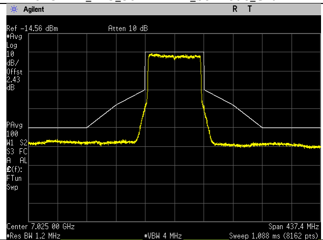
7025MHz_215_80MHz BW_be-mode_Chain 3
