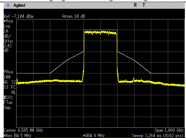
6585MHz_127_320MHz BW_be-mode_Chain 1
