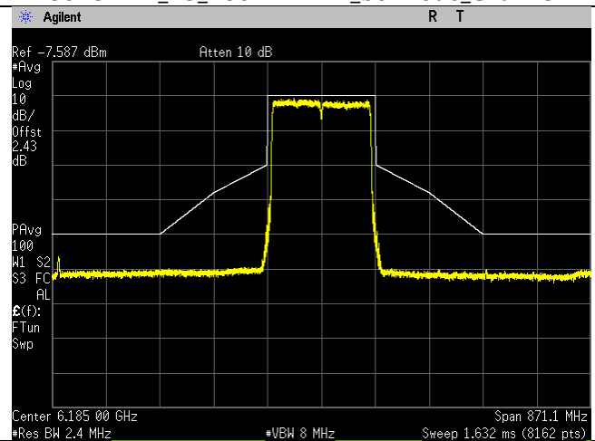
6185MHz_47_160MHz BW_be-mode_Chain 1
