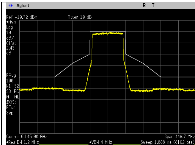
6145MHz_39_80MHz BW_be-mode_Chain 2
