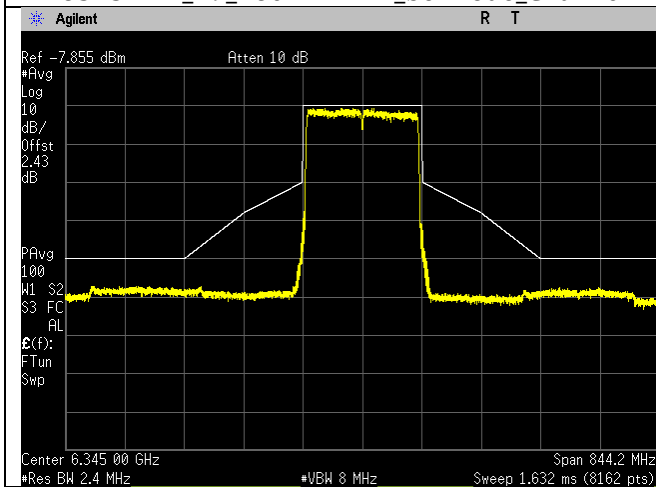
6345MHz_79_160MHz BW_be-mode_Chain 2
