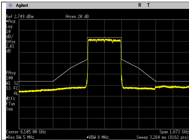
6105MHz_31_320MHz BW_be-mode_Chain 2
