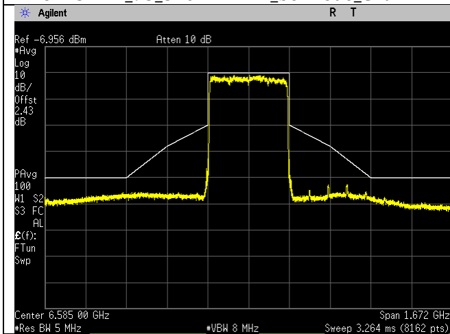
6585MHz_127_320MHz BW_be-mode_Chain 0
