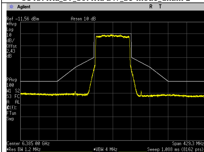
6385MHz_87_80MHz BW_be-mode_Chain 0
