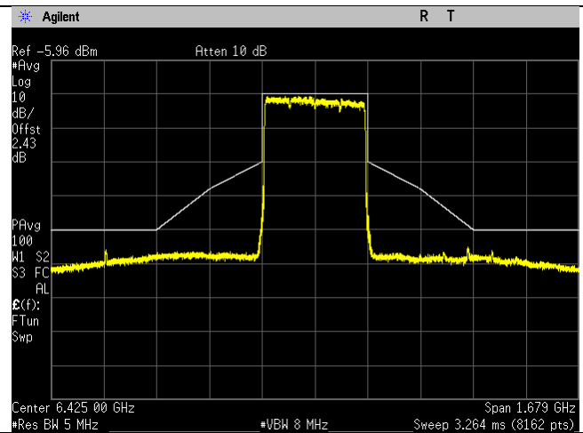
6425MHz_95_320MHz BW_be-mode_Chain 1
