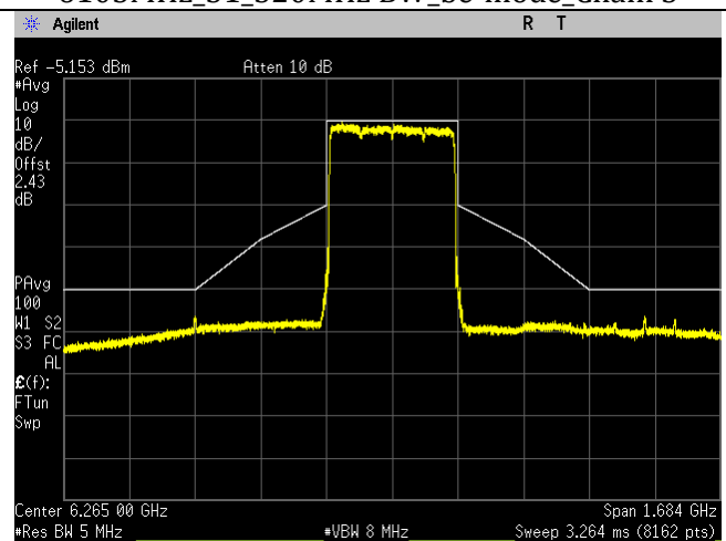
6265MHz_63_320MHz BW_be-mode_Chain 1
