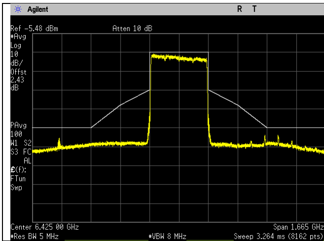
6425MHz_95_320MHz BW_be-mode_Chain 0
