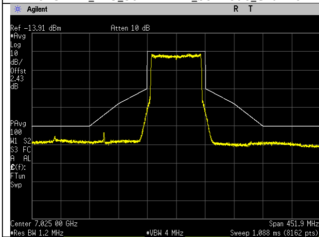
7025MHz_215_80MHz BW_be-mode_Chain 2
