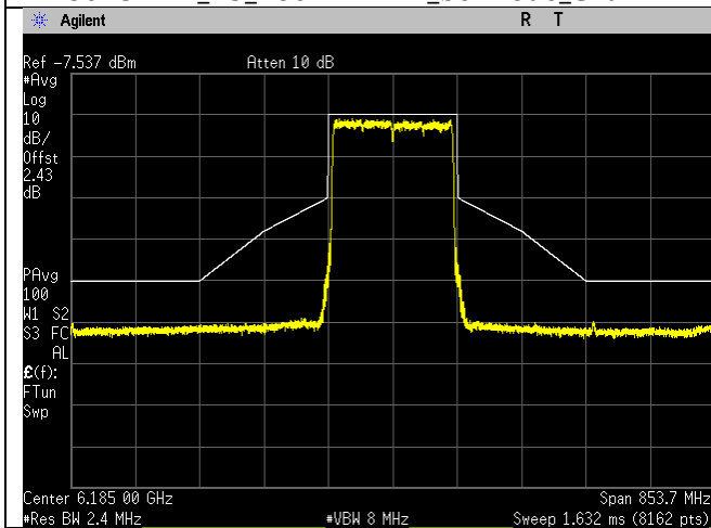
6185MHz_47_160MHz BW_be-mode_Chain 0
