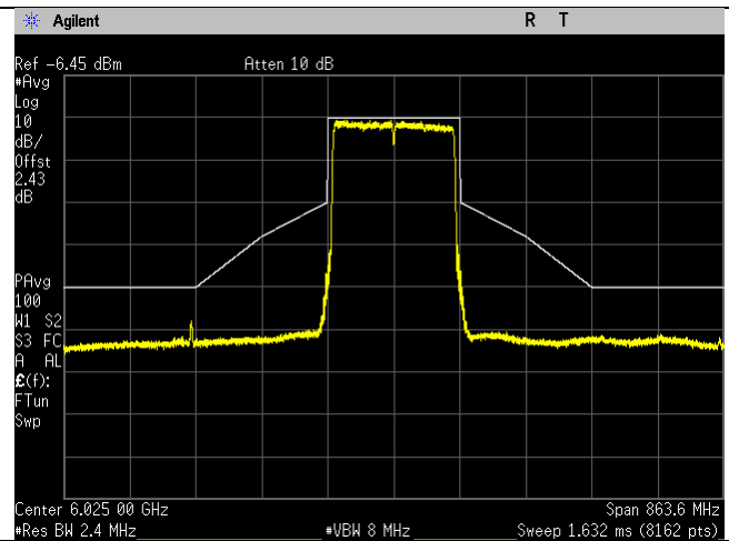
6025MHz_15_160MHz BW_be-mode_Chain 1
