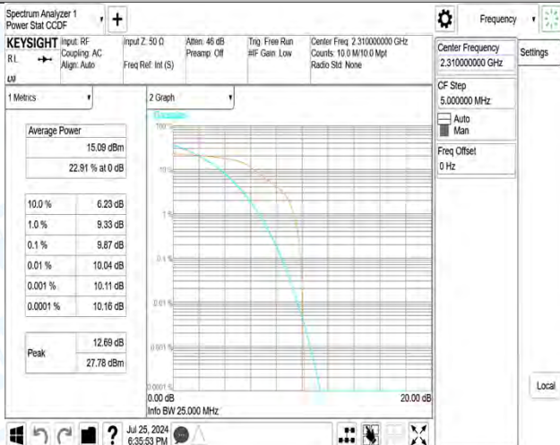
40(2305-2315)-5MHz-QPSK-38775-1RB#0-PASS
