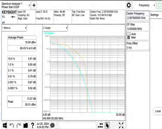
40(2305-2315)-5MHz-QPSK-38750-1RB#0-PASS
