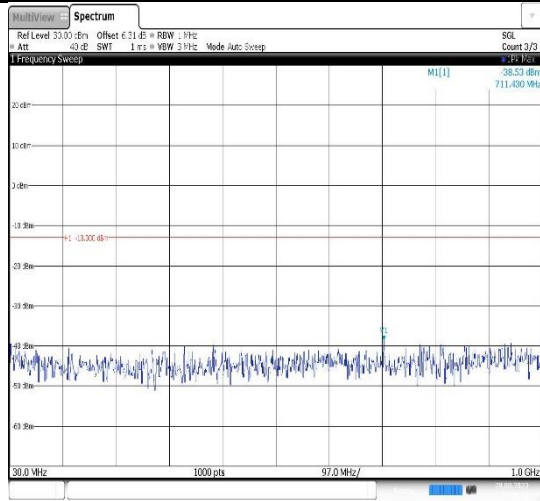
Band4-3MHz-QPSK-19965-1RB#0- Range1:30~1000MHz
