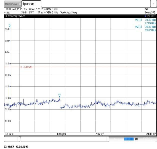
Band4-10MHz-QPSK-20175-1RB#0- Range2:1000~20000MHz
