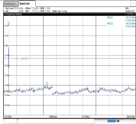
Band4-20MHz-QPSK-20175-1RB#0- Range2:1000~20000MHz
