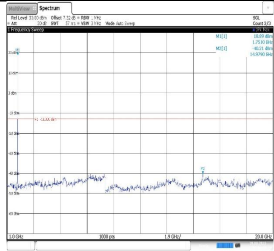
Band4-3MHz-QPSK-19965-1RB#0- Range2:1000~20000MHz
