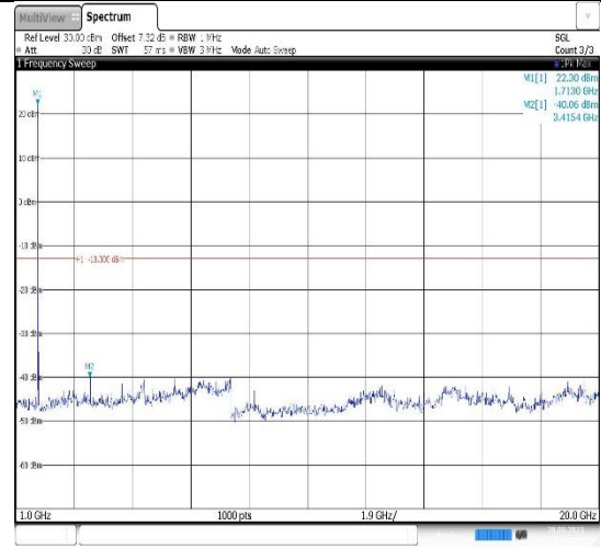
Band4-15MHz-QPSK-20025-1RB#0- Range2:1000~20000MHz
