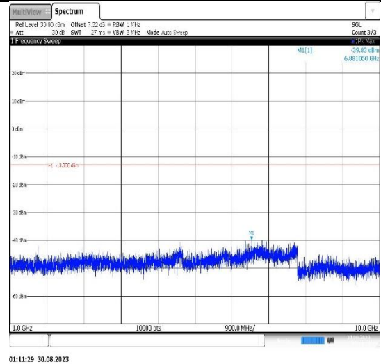
Band5-5MHz-QPSK-20425-1RB#0- Range2:1000~10000MHz
