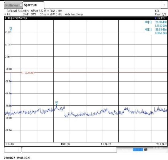
Band4-10MHz-QPSK-20000-1RB#0- Range2:1000~20000MHz
