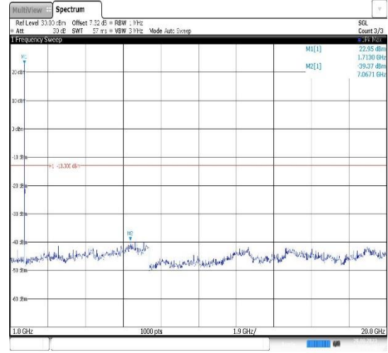
Band4-20MHz-QPSK-20050-1RB#0- Range2:1000~20000MHz
