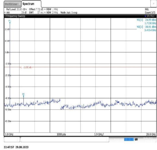
Band4-5MHz-QPSK-20175-1RB#0- Range2:1000~20000MHz
