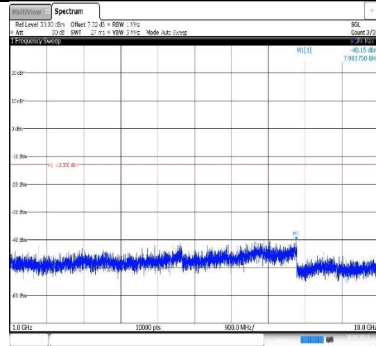
Band5-3MHz-QPSK-20415-1RB#0- Range2:1000~10000MHz
