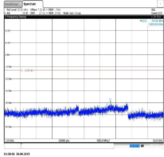
Band5-5MHz-QPSK-20525-1RB#0- Range2:1000~10000MHz
