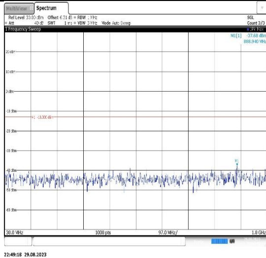
Band4-10MHz-QPSK-20000-1RB#0- Range1:30~1000MHz
