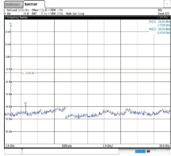
Band4-3MHz-QPSK-20175-1RB#0- Range2:1000~20000MHz
