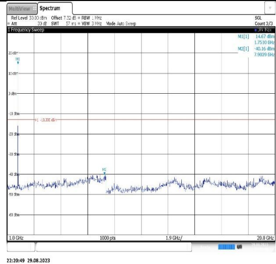
Band4-5MHz-QPSK-19975-1RB#0- Range2:1000~20000MHz
