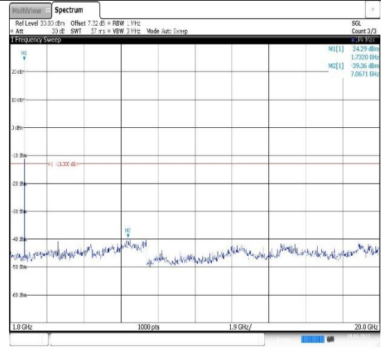
Band4-3MHz-QPSK-20385-1RB#0- Range2:1000~20000MHz
