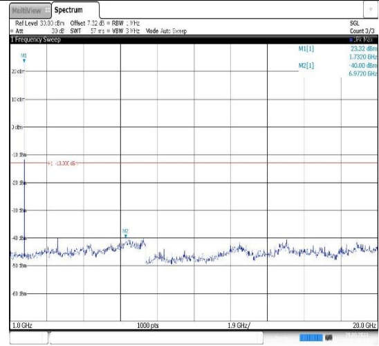
Band4-1.4MHz-QPSK-20175-1RB#0- Range2:1000~20000MHz
