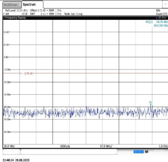
Band4-5MHz-QPSK-20375-1RB#0- Range1:30~1000MHz
