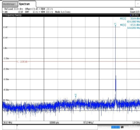
Band5-3MHz-QPSK-20415-1RB#0- Range1:30~1000MHz
