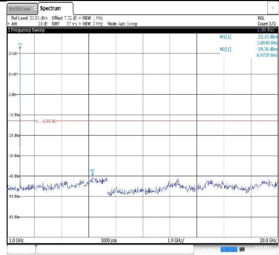
Band4-1.4MHz-QPSK-19957-1RB#0- Range2:1000~20000MHz
