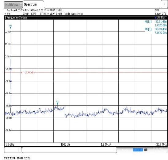
Band4-10MHz-QPSK-20350-1RB#0- Range2:1000~20000MHz
