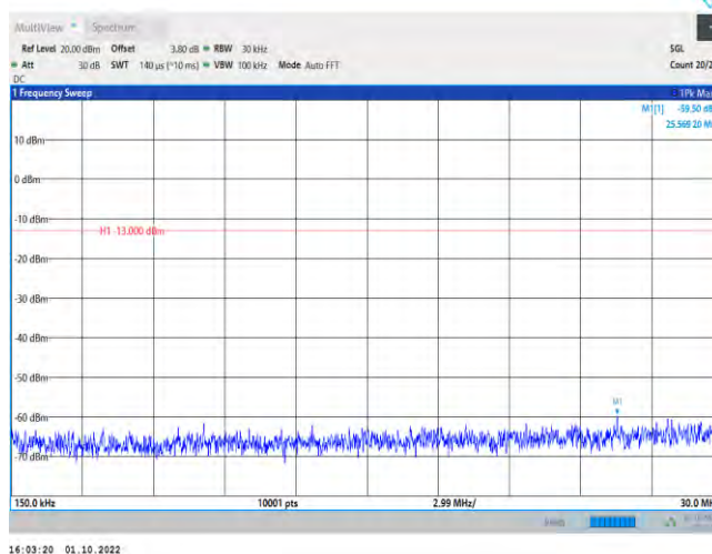
GSM850-128-0.15~30MHz
