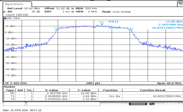
11G-CDD_Ant7_2462
