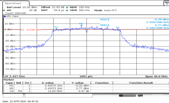
11G-CDD_Ant6_2437
