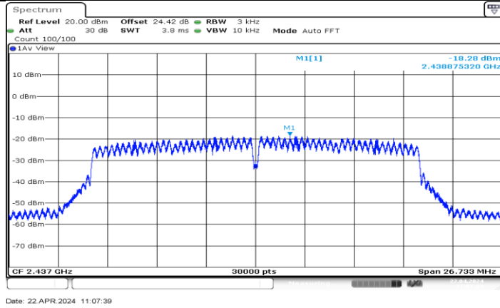
11N20MIMO_Ant7_2437
