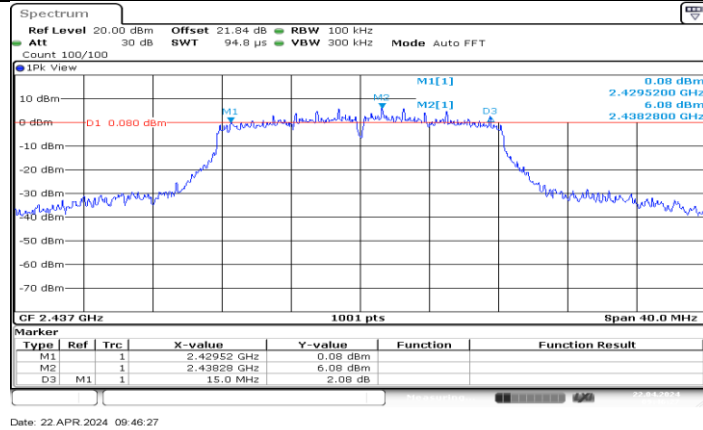
11G-CDD_Ant7_2437
