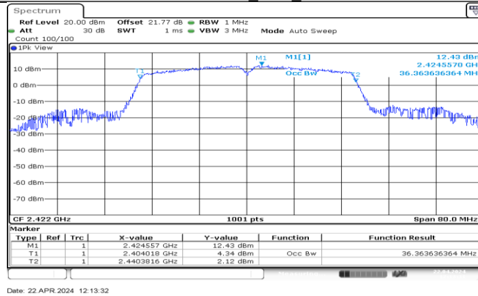
11N40MIMO_Ant7_2422
