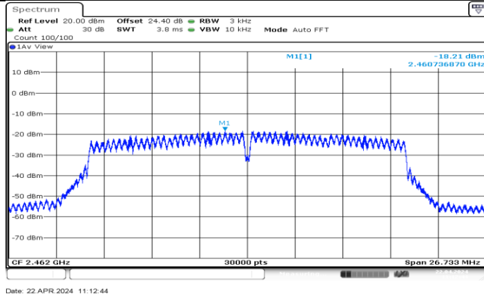
11N20MIMO_Ant7_2462
