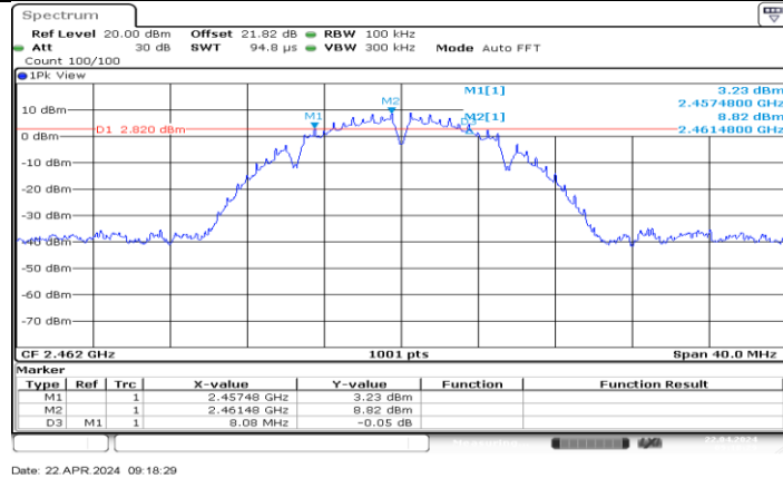
11B-CDD_Ant7_2462
