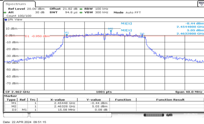
11G-CDD_Ant7_2462
