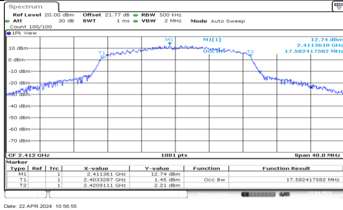
11N20MIMO_Ant7_2412
