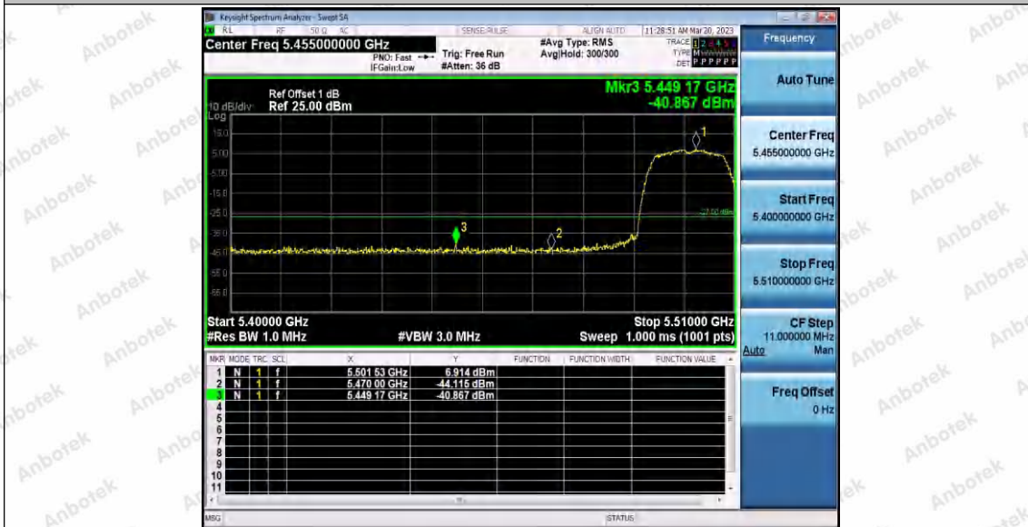
11A_Ant2_Low_5500
