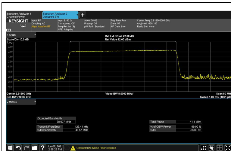
Figure 167: output 256QAM 40MHz B.W.; 2516.0MHz, 15kHz
