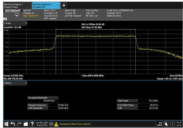
Figure 190: output QPSK 40MHz B.W.; 2670.0MHz, 60kHz
