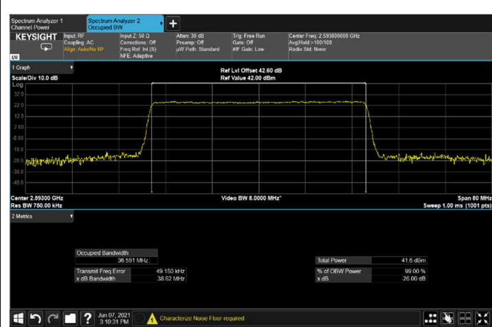
Figure 172: output 256QAM 40MHz B.W.; 2593.0MHz, 60kHz
