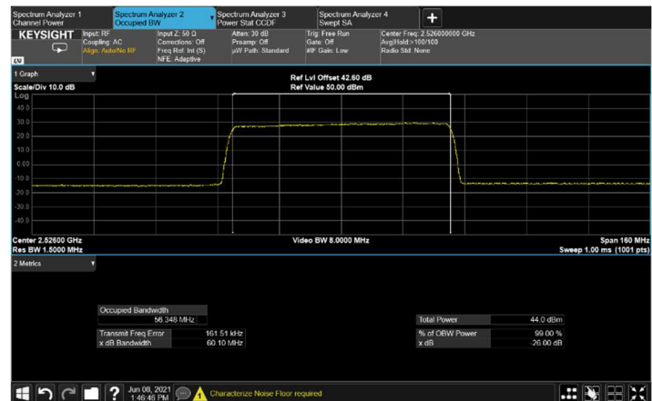
Figure 162: output 64QAM 60MHz B.W.; 2526.0MHz, 60kHz
