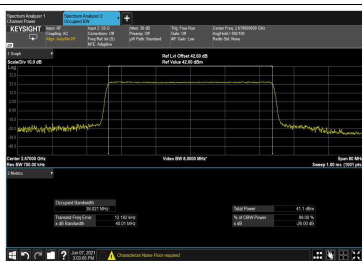
Figure 174: output 256QAM 40MHz B.W.; 2670.0MHz, 30kHz
