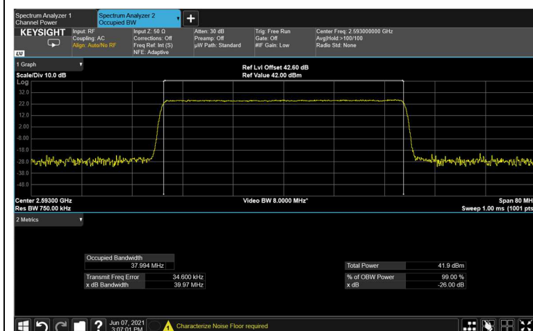
Figure 171: output 256QAM 40MHz B.W.; 2593.0MHz, 30kHz
