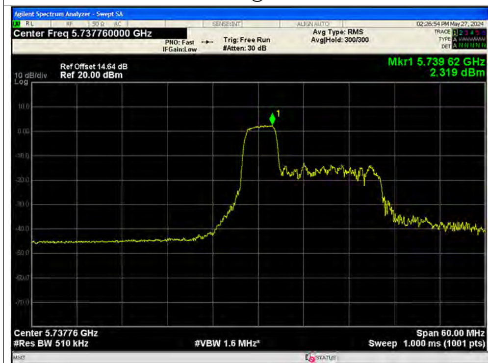
PSD NVNT ax40 52@37 5755MHz Ant2
