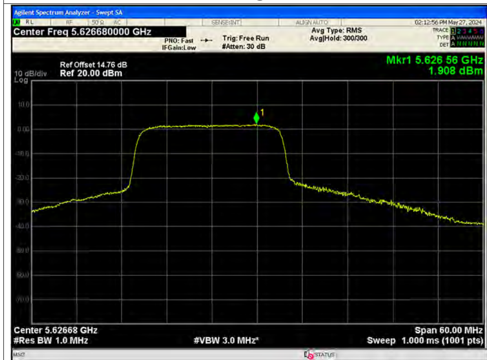
PSD NVNT ax40 242@61 5630MHz Ant1
