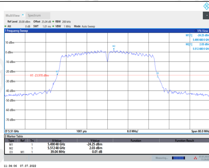
11N40MIMO_Ant2_5510
