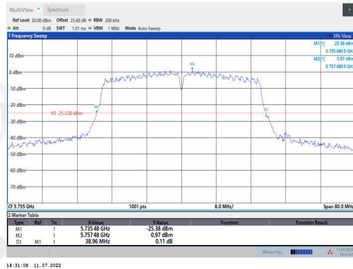
11AC40MIMO_Ant2_5755
