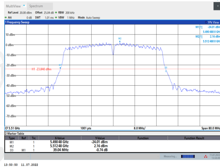
11AC40MIMO_Ant2_5510
