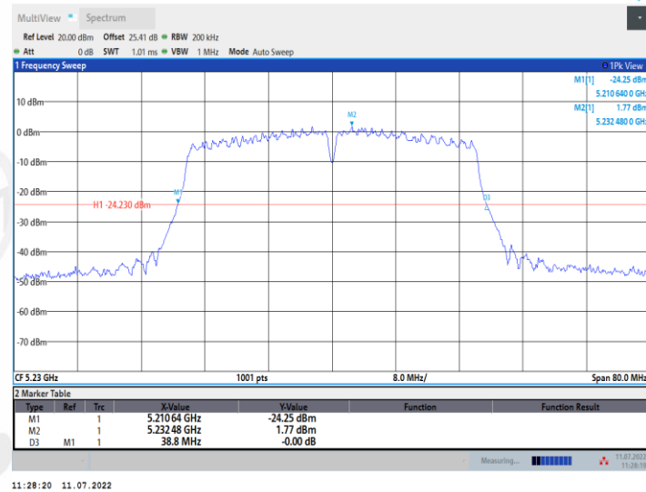
11AC40MIMO_Ant2_5230
