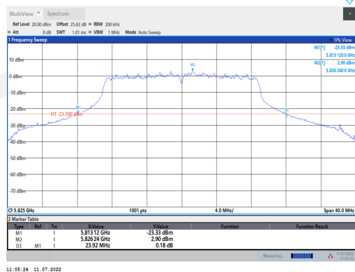
11AC20MIMO_Ant2_5825
