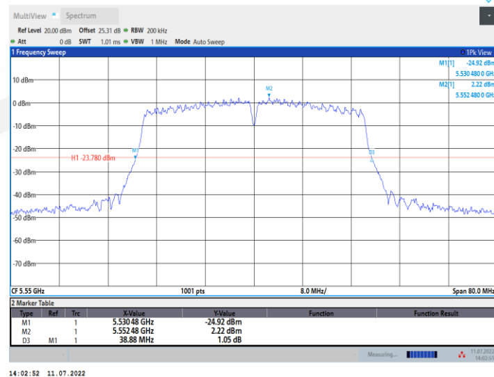
11AC40MIMO_Ant2_5550
