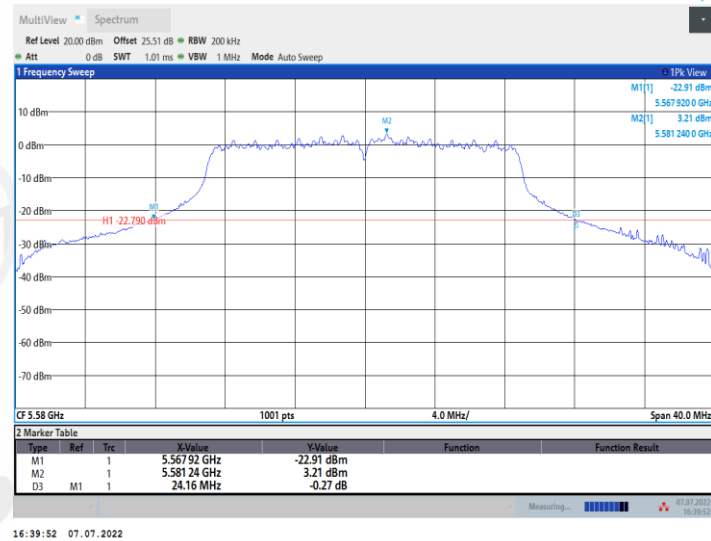
11AC20MIMO_Ant2_5580
