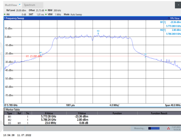
11AC20MIMO_Ant2_5785
