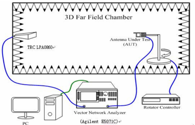
图. 1. 微波暗室内仪器设置 r.4
