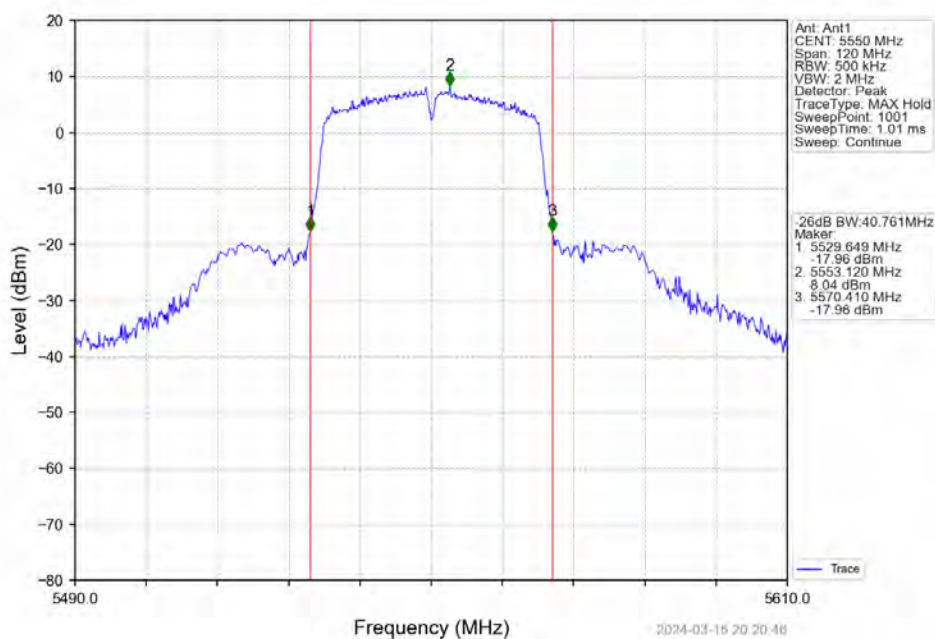
802.11n(HT40) MCH_5550MHz_Ant7_NTNV
