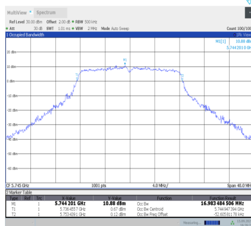
11a-Ant1-5745
