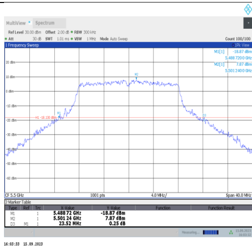
11a-Ant1-5500
