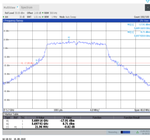
11a-Ant1-5700
