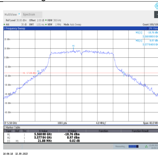
11a-Ant1-5580
