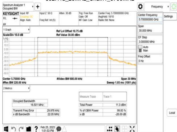
802.11a_20MHz_Chain1_5700MHz
