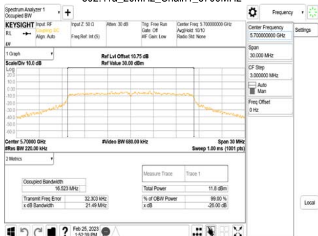
802.11a_20MHz_Chain1_5700MHz
