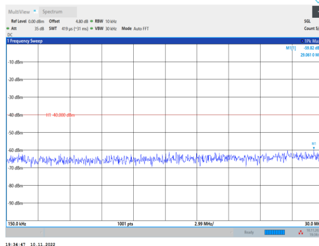
Band48-20MHz-QPSK-55340-1RB#0-Range2:0.15~30MHz
