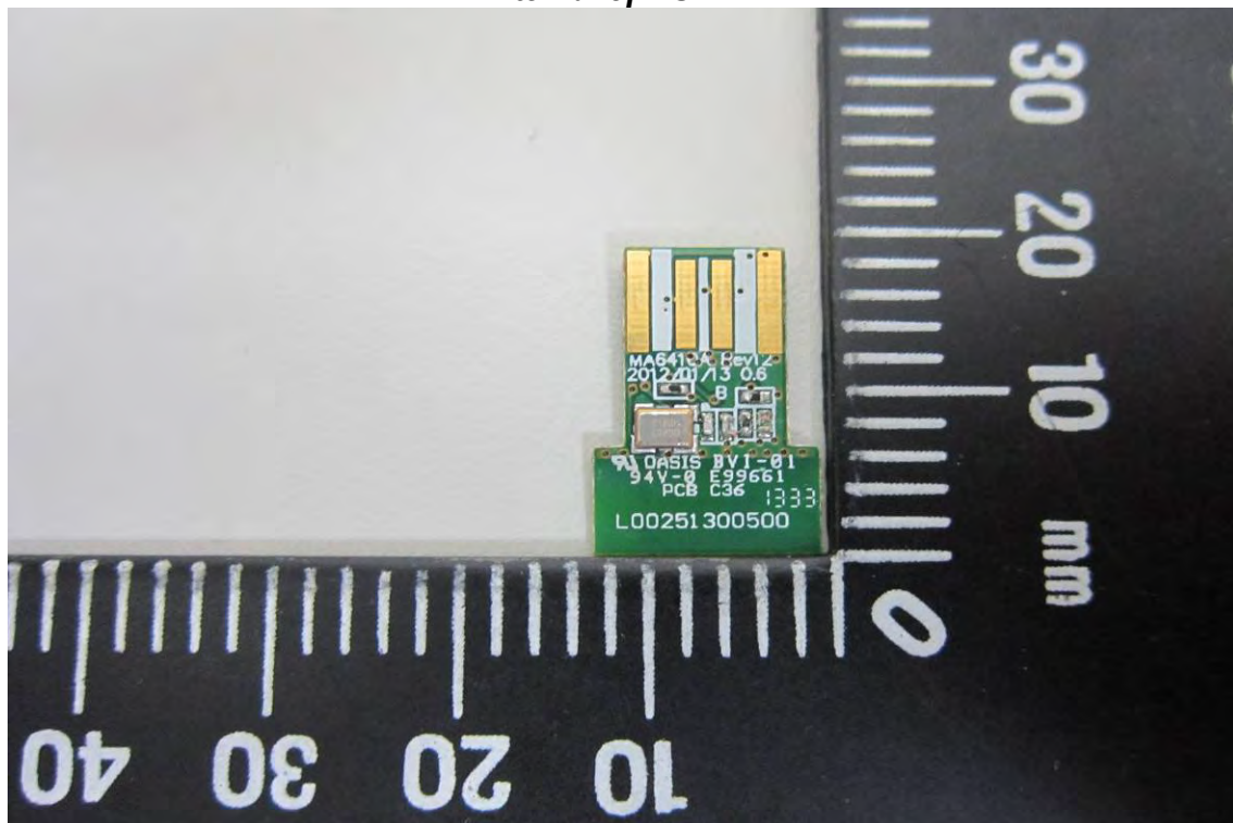
2.4GHz Antenna
