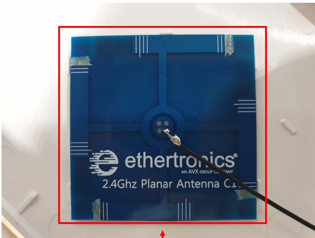
Antenna 3(TX, RX)(Freq : 2402-2480 MHz)
