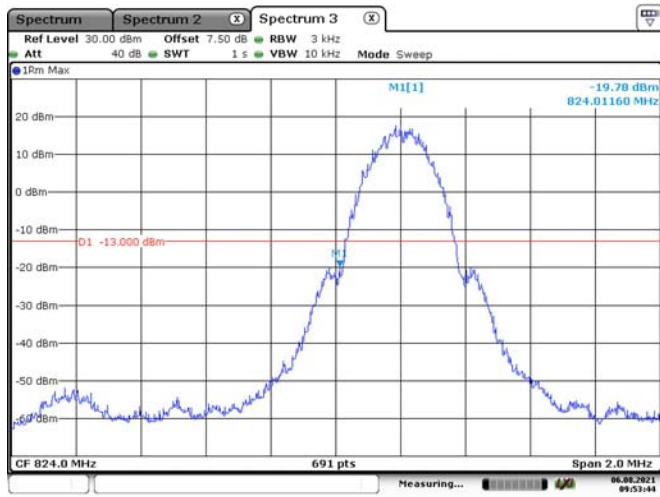
GPRS 850, Left Band Edge
