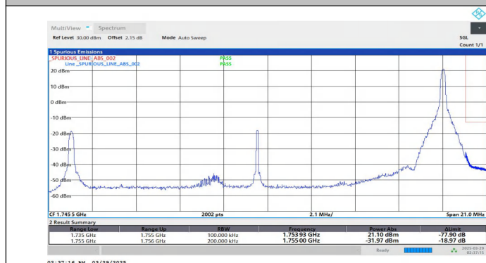
Band4-20MHz-QPSK-20300-1RB#99-PASS
