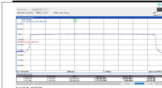
Band4-20MHz-QPSK-20050-100RB#0-PASS
