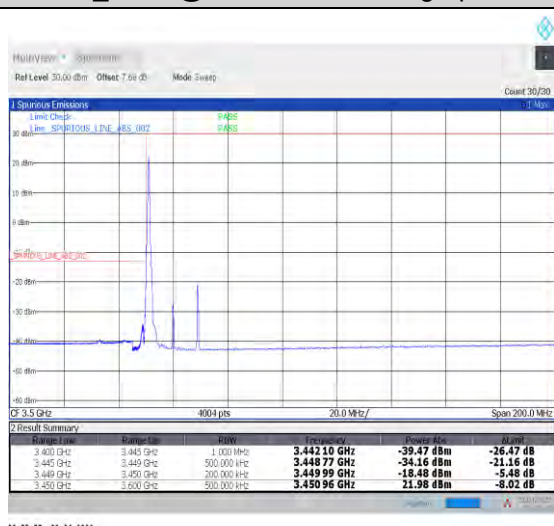
1-N78-3450-3550--30-20-L-4-CP-QPSK-Edge_1RB_L eft-1@0-Ant0-PASS-see graph
