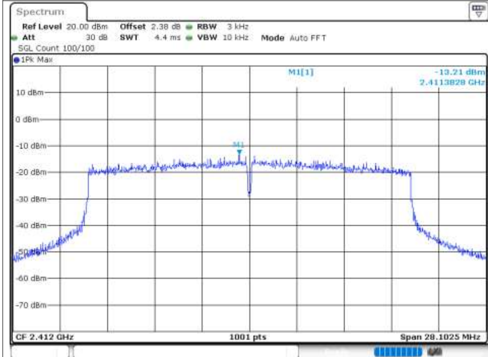
PSD NVNT ax20 2412MHz Ant1
