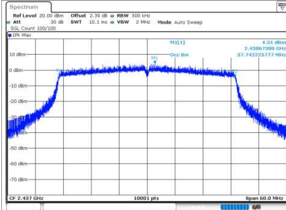
OBW NVNT ax40 2437MHz Ant1
