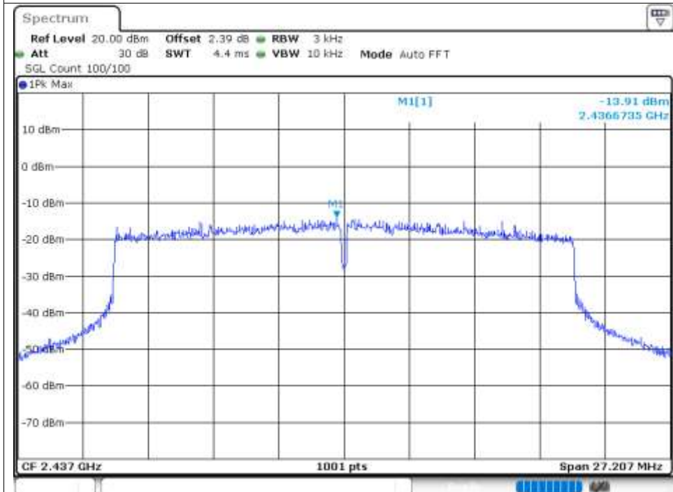
PSD NVNT ax20 2437MHz Ant1
