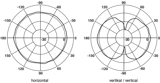
Richtcharakteristik / Radiation pattern / Diagramme de rayonnement / Característica direccional
