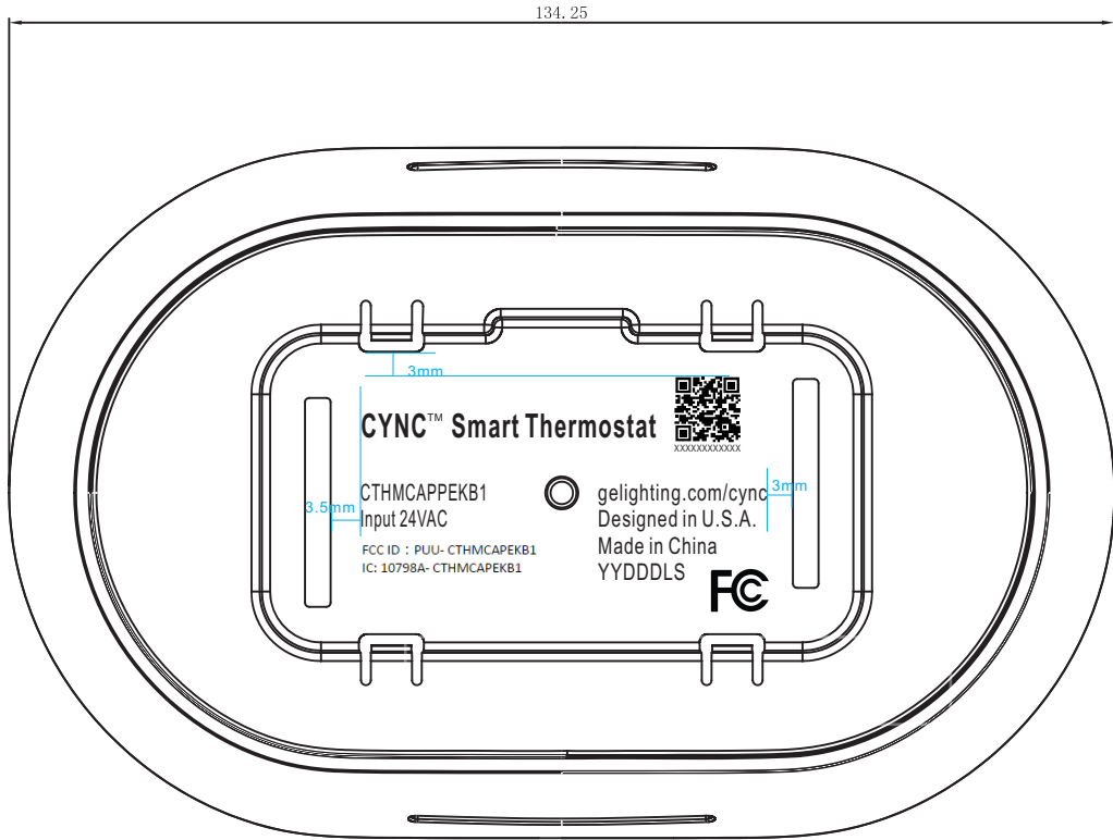
后壳
