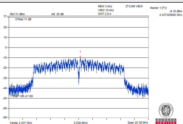
802.11g : CH 6
