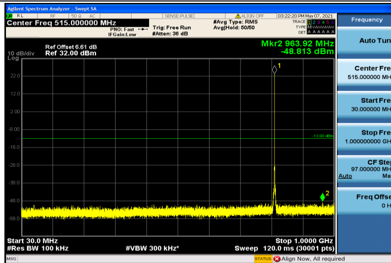
Band26-1.4MHz-QPSK-26697-1RB#0-30~1000MHz
