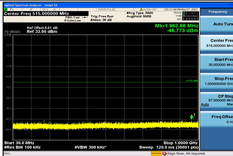
Band25-20MHz-QPSK-26140-1RB#0-30~1000MHz
