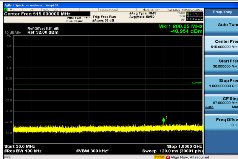
Band25-1.4MHz-QPSK-26365-1RB#0-30~1000MHz
