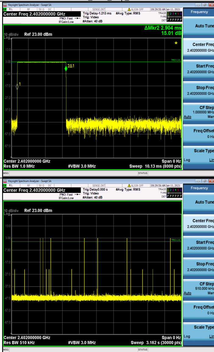
DH5_Ant1_Hop_2402
