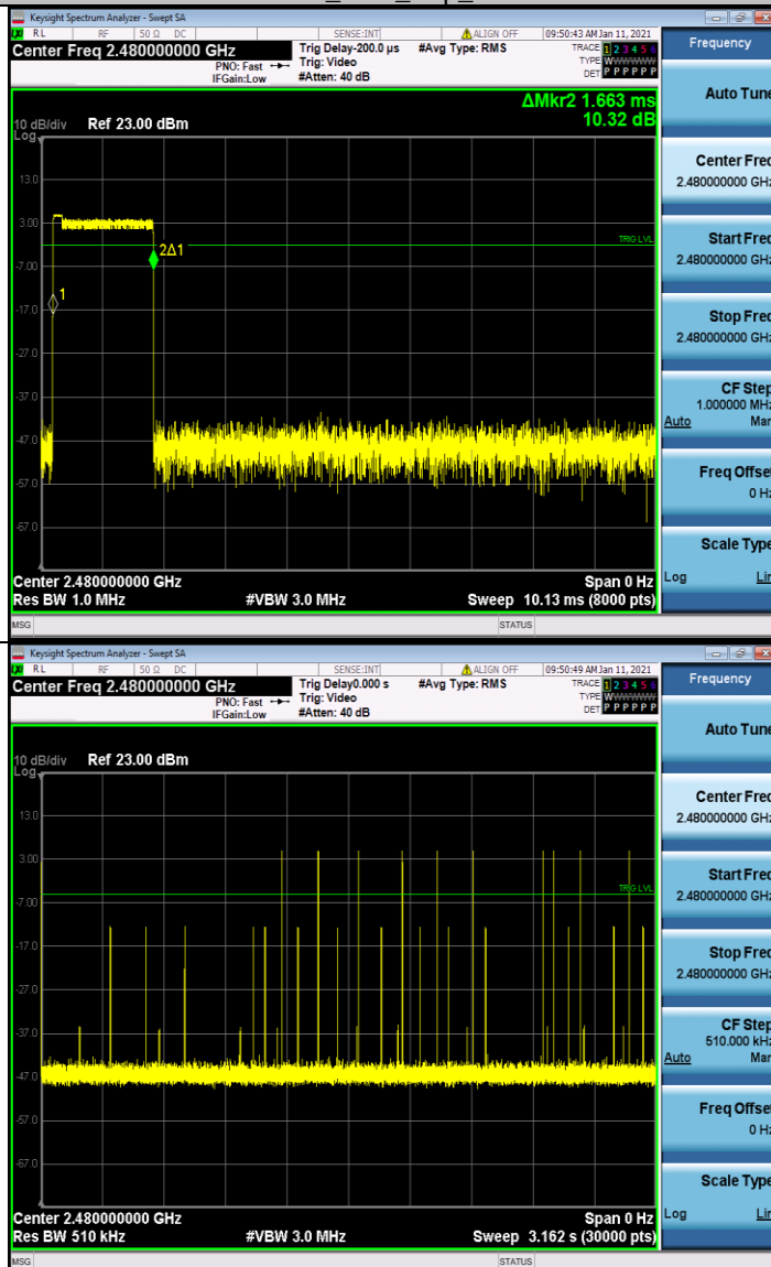
2DH3_Ant1_Hop_2480
