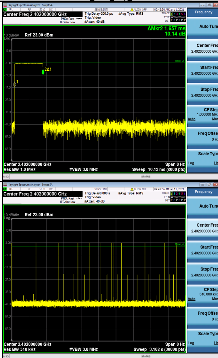
DH3_Ant1_Hop_2402
