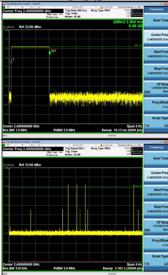
DH5_Ant1_Hop_2480
