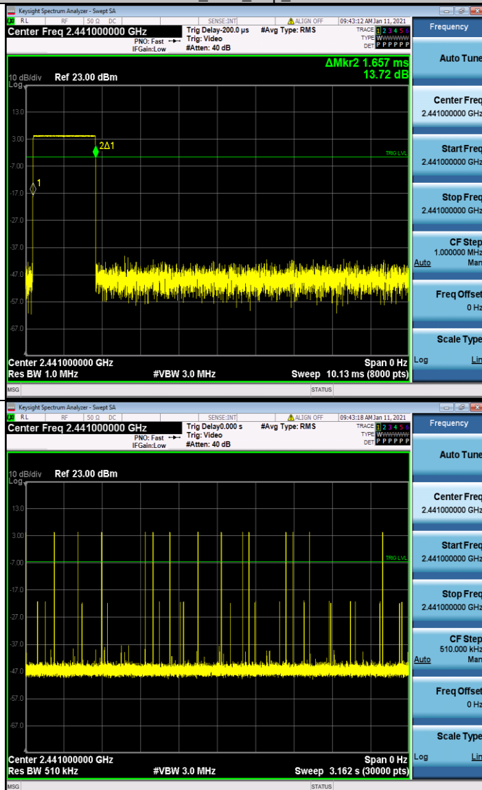
DH3_Ant1_Hop_2441
