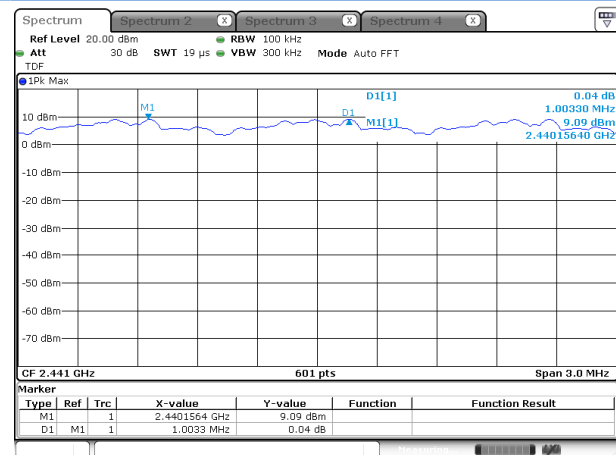
\Pi/4 -DQPSK
