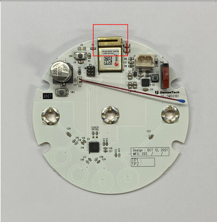
ANTENNA(2.4 GHz)
