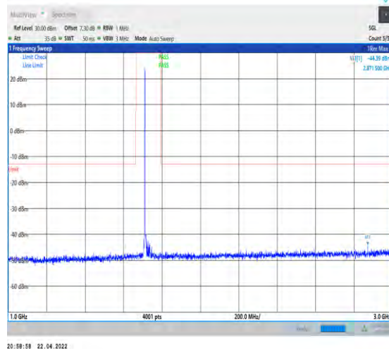
1-N66-PC3-15-40-L-1-DFT-PI2BPSK-Inner_1RB_Lef t-1@1-1000-3000-Ant0--44.39--13-PASS
