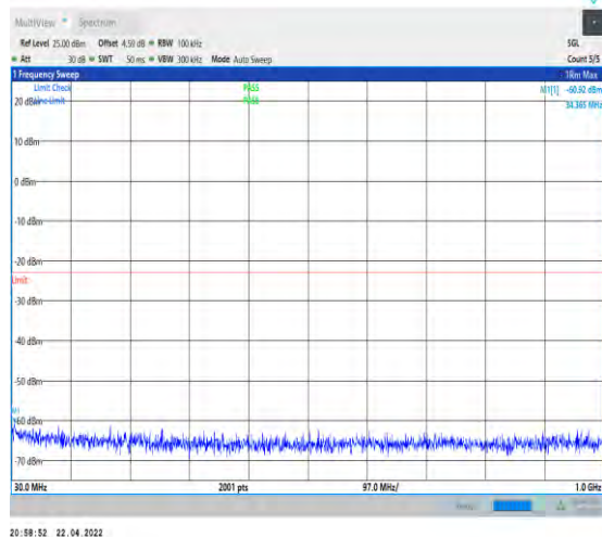
1-N66-PC3-15-40-L-1-DFT-PI2BPSK-Inner_1RB_Le ft-1@1-30-1000-Ant0--60.92--23-PASS
