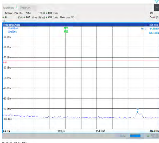
1-N66-PC3-15-40-M-1-DFT-PI2BPSK-Inner_1RB_L eft-1@1-0.009-0.15-Ant0--94.19--43-PASS
