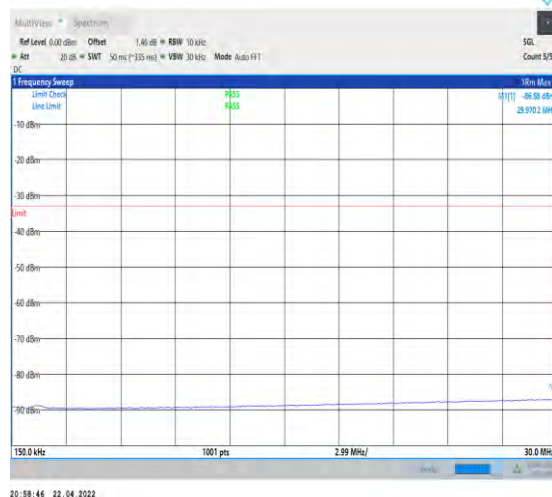
1-N66-PC3-15-40-L-1-DFT-PI2BPSK-Inner_1RB_Lef t-1@1-0.15-30-Ant0--86.88--33-PASS
