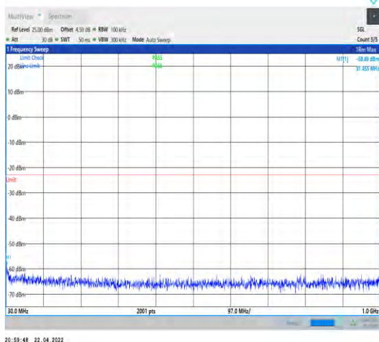
1-N66-PC3-15-40-M-1-DFT-PI2BPSK-Inner_1RB_L eft-1@1-30-1000-Ant0--58.89--23-PASS
