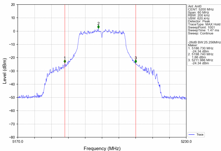
802.11a_MCH_5200MHz_Ant0_NTNV
