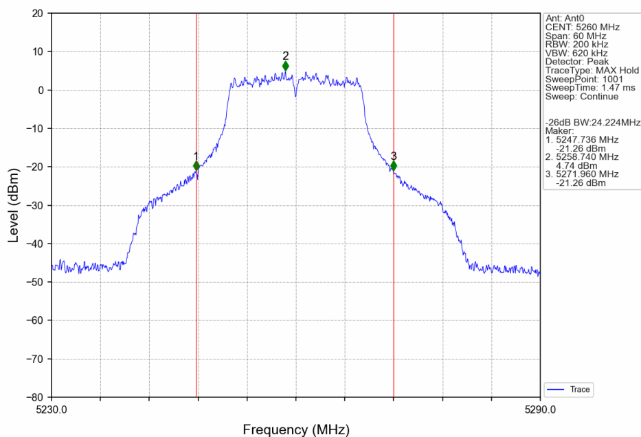
802.11a_LCH_5260MHz_Ant0_NTNV
