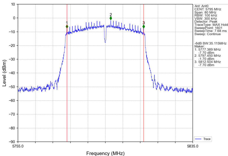
802.11n(HT40)_HCH_5795MHz_Ant0_NTNV
