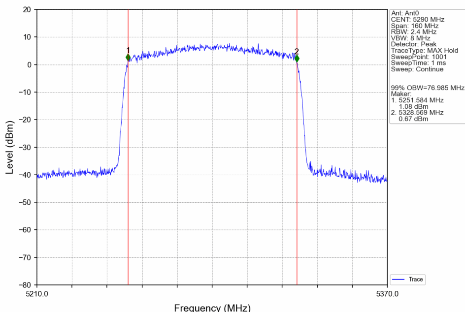
802.11ax(HEW80)_MCH_5290MHz_RU996_Left_Ant0_NTNV
