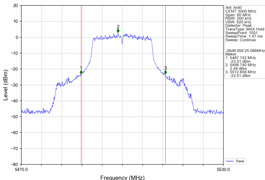
802.11n(HT20)_LCH_5500MHz_Ant0_NTNV
