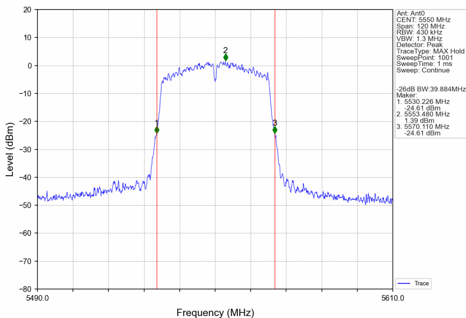
802.11n(HT40)_MCH_5550MHz_Ant0_NTNV
