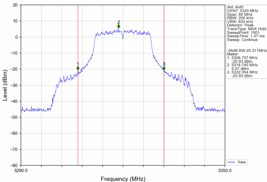
802.11a_HCH_5320MHz_Ant0_NTNV
