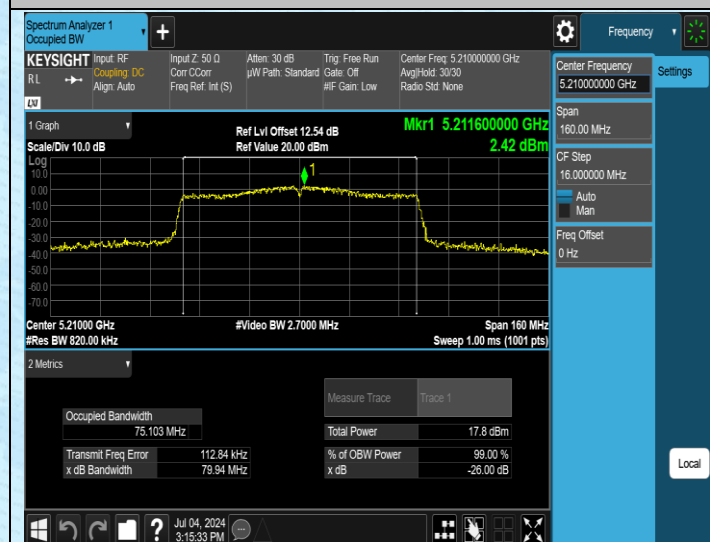
11AC80SISO-Ant1-5210
