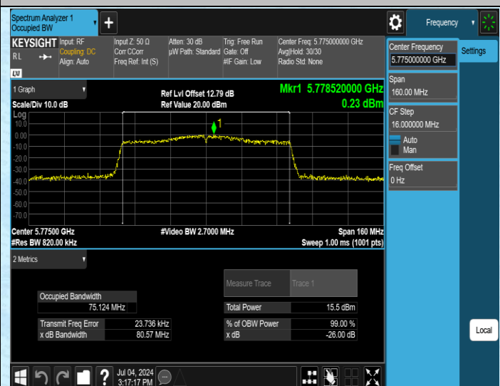
11AC80SISO-Ant1-5775
