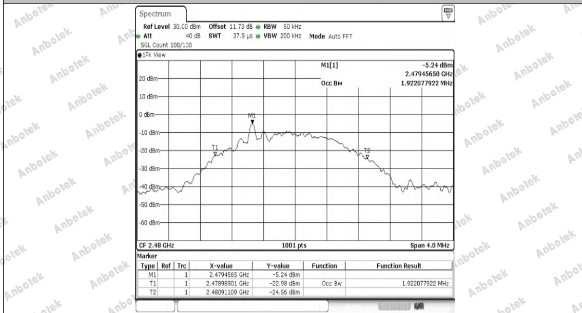
BLE_2M-Ant1-2480
