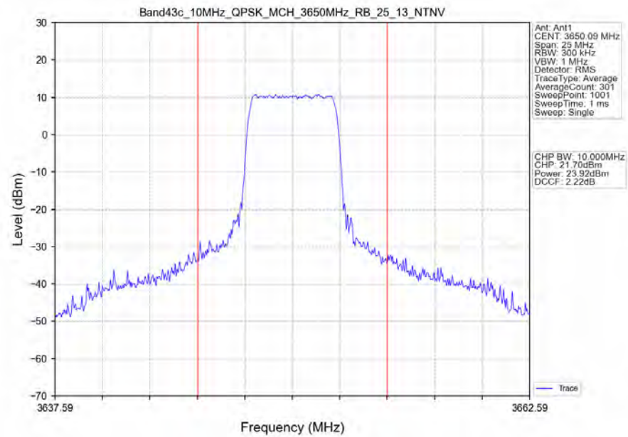
Band43c_10MHz_QPSK_MCH_3650MHz_RB_25_13_NTNV
