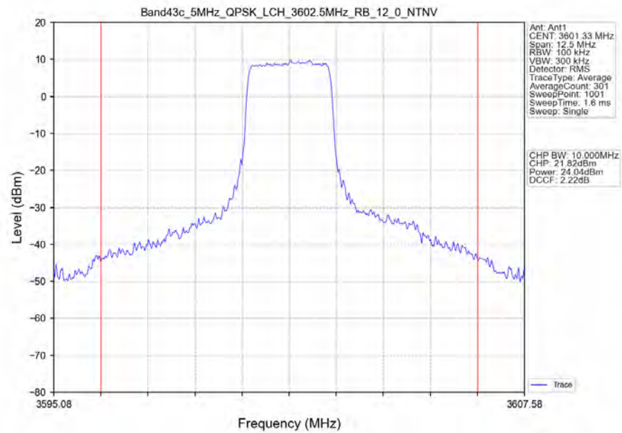
Band43c_5MHz_QPSK_LCH_3602.5MHz_RB_12_0_NTNV
