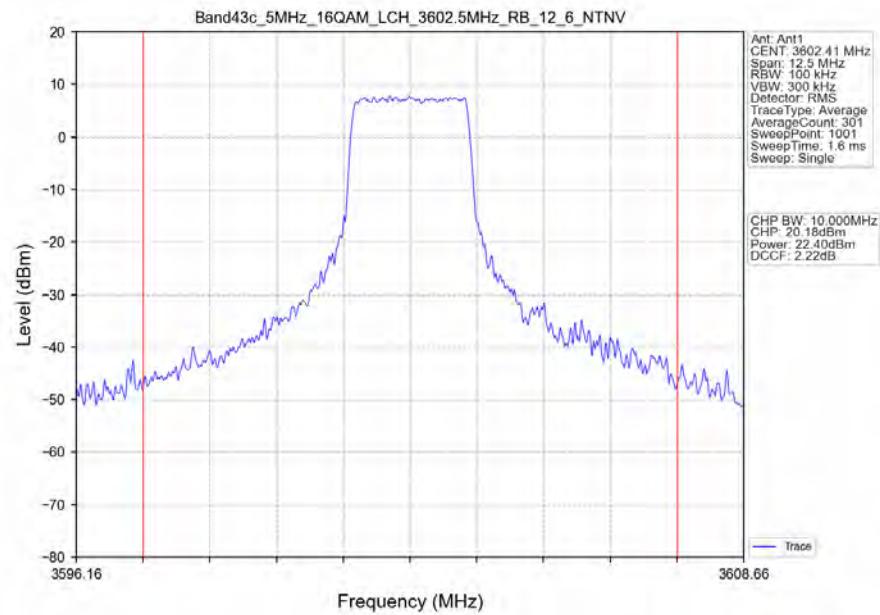
Band43c_5MHz_16QAM_LCH_3602.5MHz_RB_12_6_NTNV
