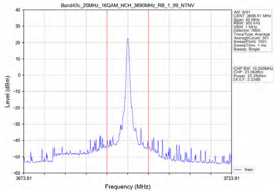
Band43c_20MHz_16QAM_HCH_3690MHz_RB_1_99_NTNV
