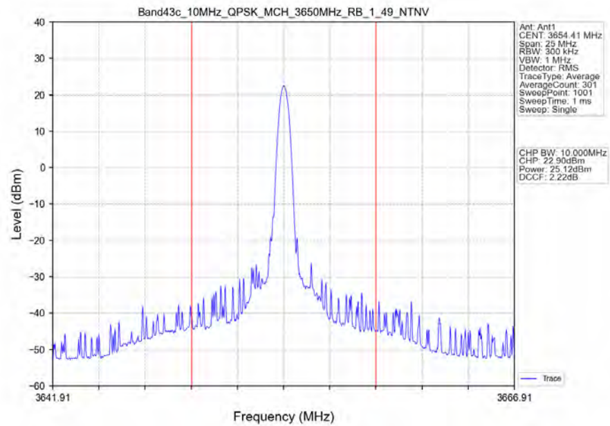
Band43c_10MHz_QPSK_MCH_3650MHz_RB_1_49_NTNV
