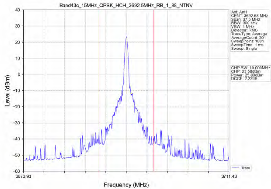
Band43c_15MHz_QPSK_HCH_3692.5MHz_RB_1_38_NTNV
