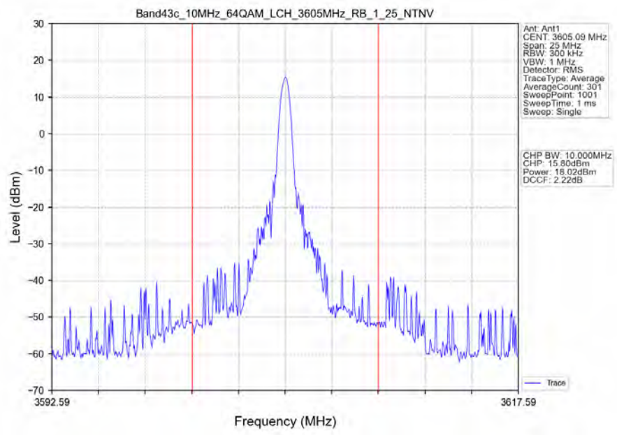
Band43c_10MHz_64QAM_LCH_3605MHz_RB_1_25_NTNV
