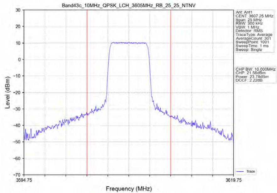
Band43c_10MHz_QPSK_LCH_3605MHz_RB_25_25_NTNV
