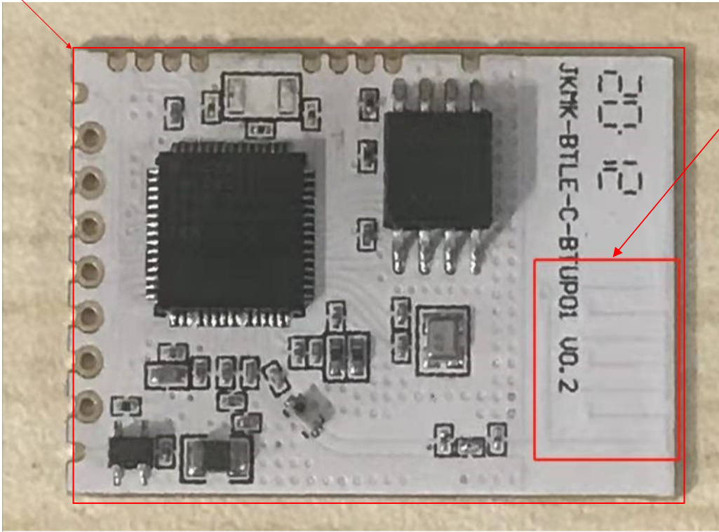
RF Module
