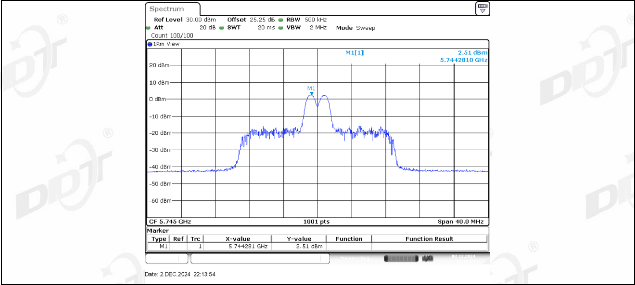
11AX20MIMO_Ant2_5745_26Tone_RU5
