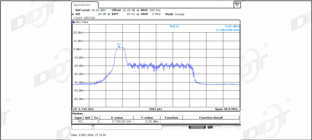
11AX20MIMO_Ant2_5745_26Tone_RU4
