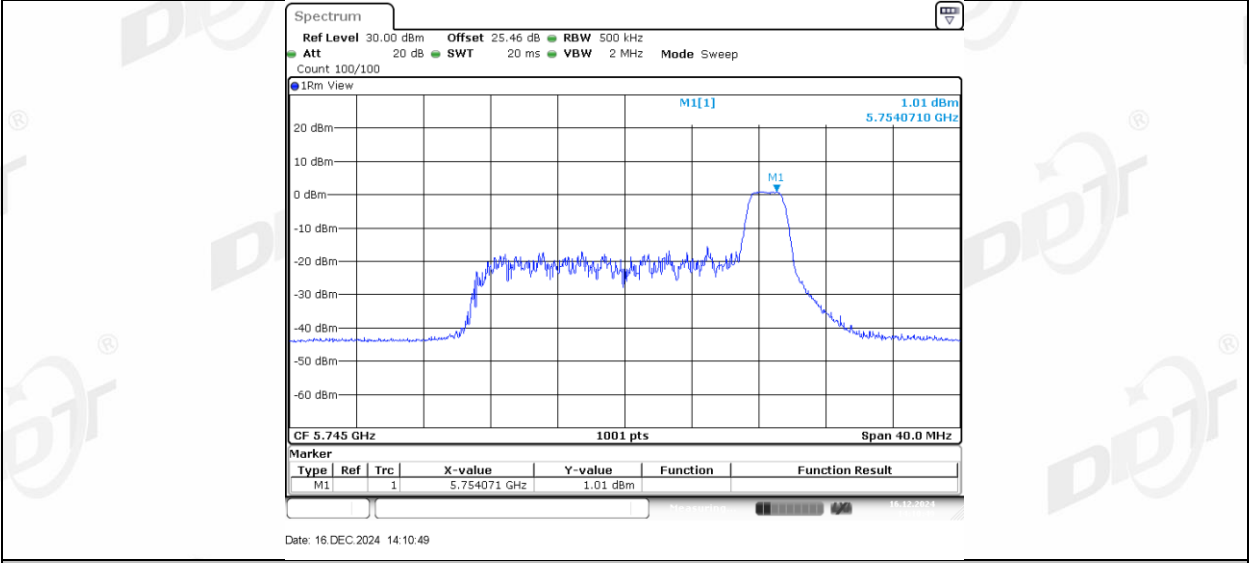
11AX20MIMO_Ant2_5745_52Tone_RU37
