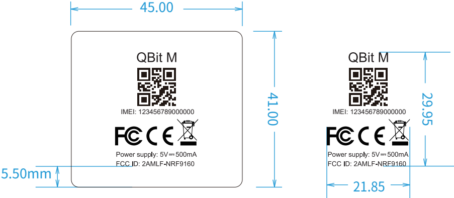
产品背面镭雕 IMEI根据产品信息表更新, 每个产品对应不同的IMEI号码
