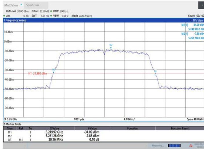
11AC20MIMO_Ant2_5260
