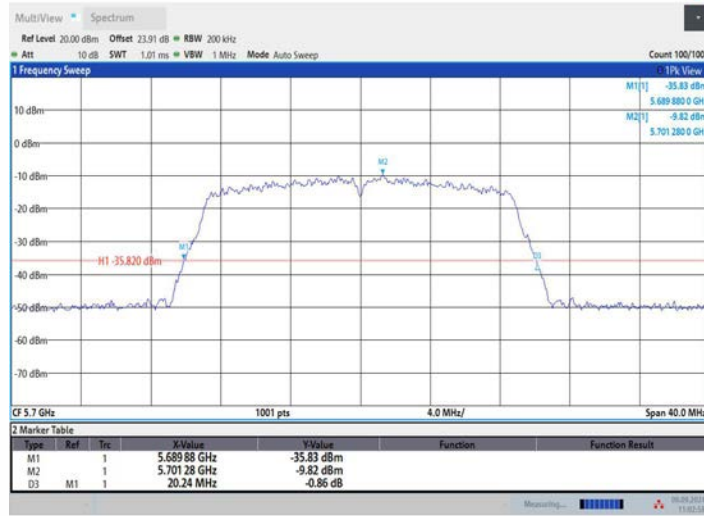
11AC20MIMO_Ant2_5700
