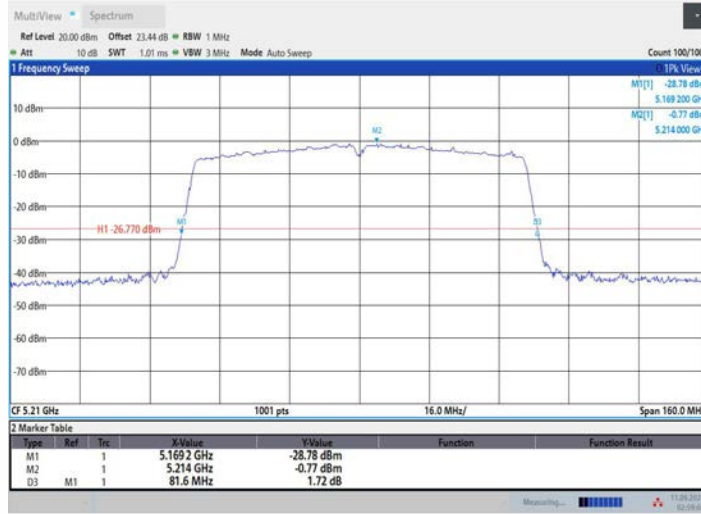
11AC80MIMO_Ant2_5210
