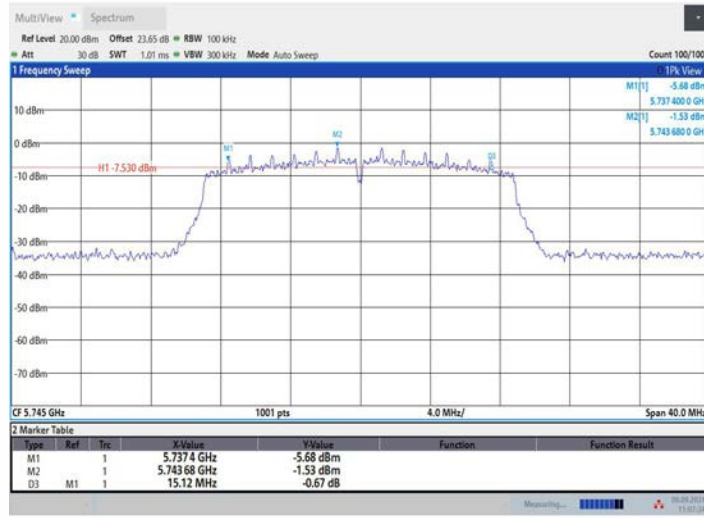
11AC20MIMO_Ant2_5745
