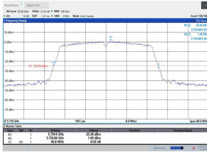
11AC40MIMO_Ant2_5755
