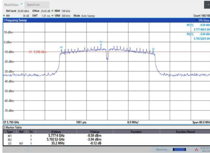
11N40MIMO_Ant2_5795
