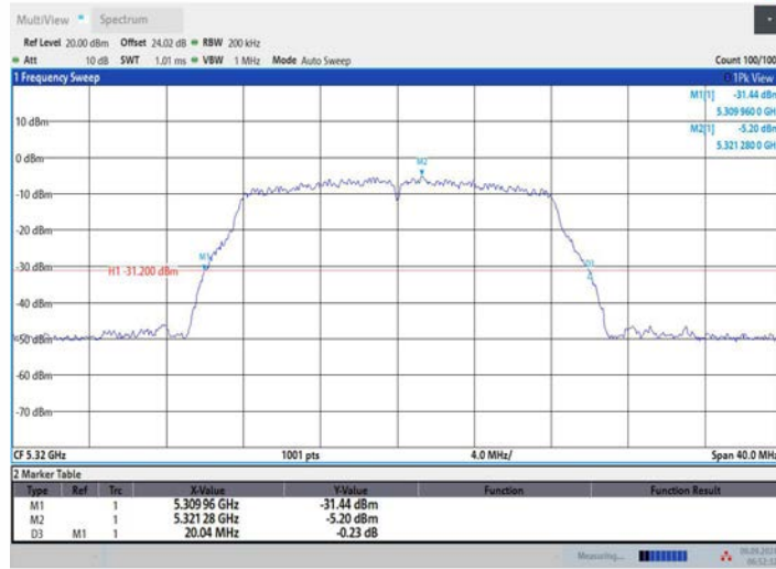
11A_Ant2_5320
