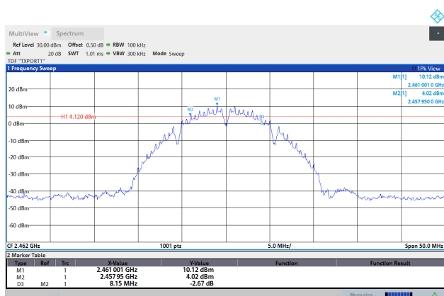
802.11b / 2 462 MHz
