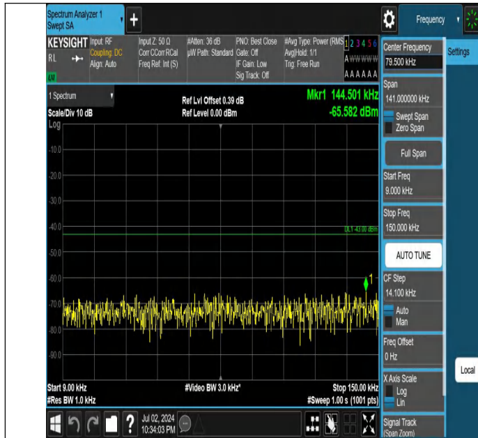
Band4-20MHz-QPSK-20175-1RB#0-0.009~0.15-PASS
