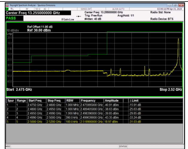
Band7_20MHz_QPSK_20850_1RB#99
