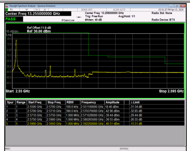
Band7_20MHz_16QAM_21350_1RB#0
