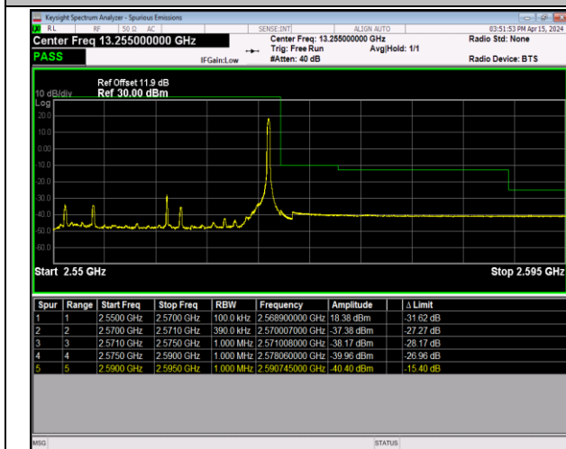
Band7_20MHz_16QAM_21350_1RB#99
