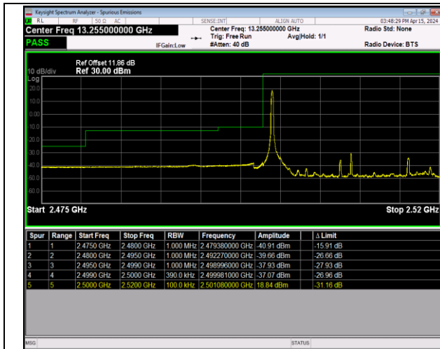
Band7_20MHz_QPSK_20850_1RB#0
