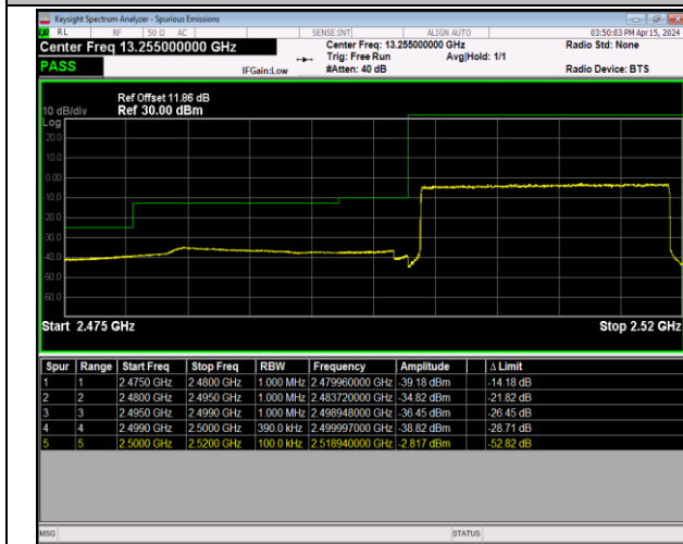
Band7_20MHz_QPSK_20850_100RB#0
