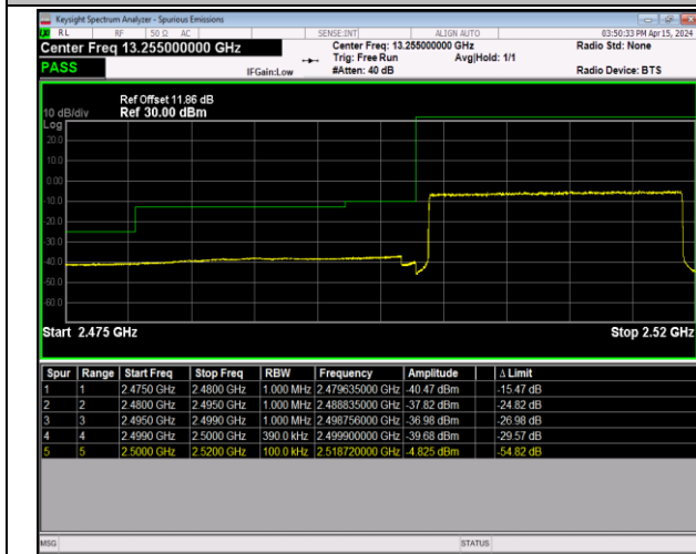
Band7_20MHz_64QAM_20850_100RB#0
