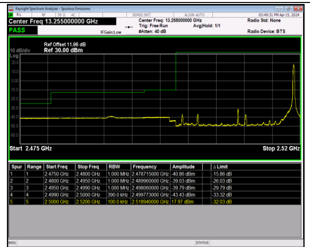
Band7_20MHz_16QAM_20850_1RB#99
