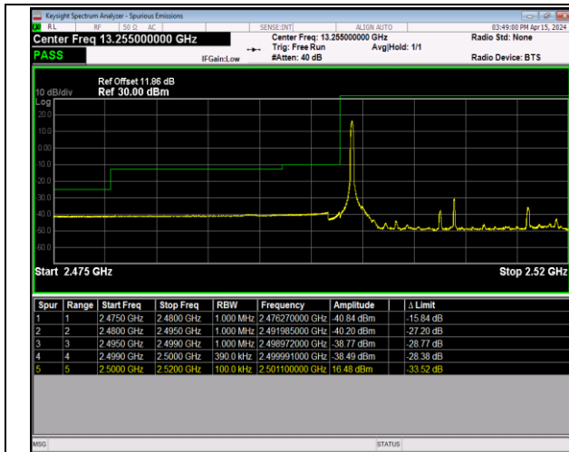
Band7_20MHz_64QAM_20850_1RB#0
