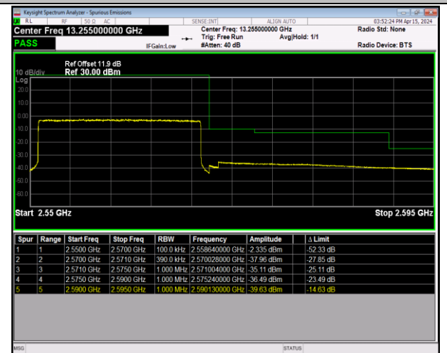
Band7_20MHz_QPSK_21350_100RB#0
