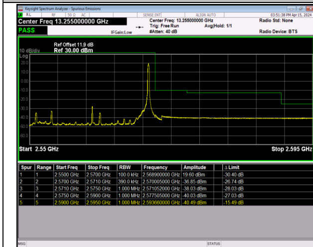
Band7_20MHz_QPSK_21350_1RB#99
