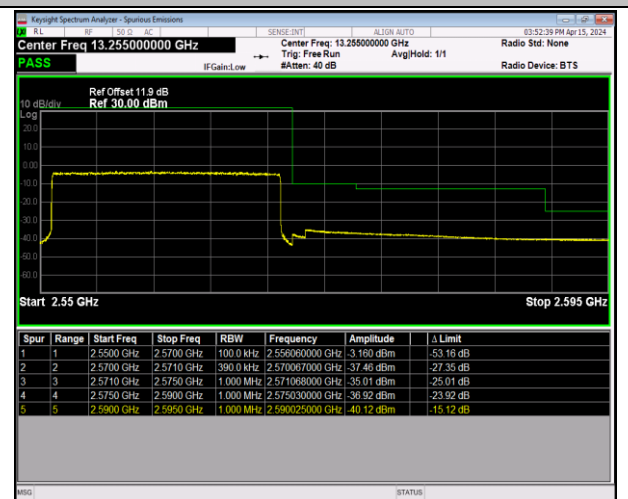
Band7_20MHz_16QAM_21350_100RB#0
