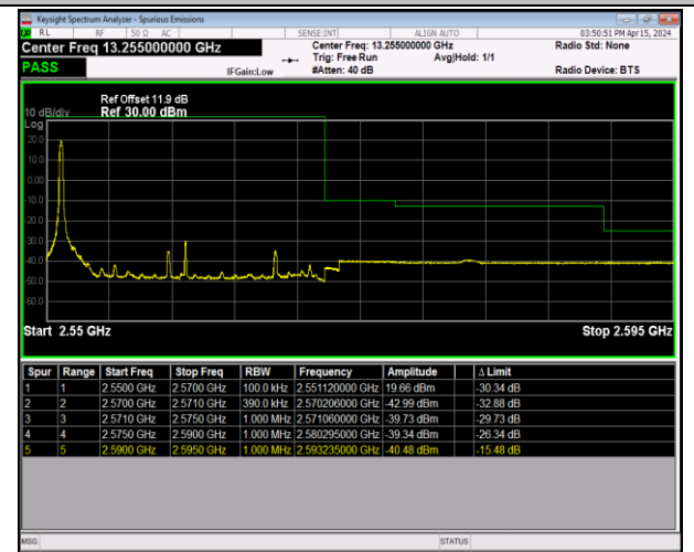
Band7_20MHz_QPSK_21350_1RB#0
