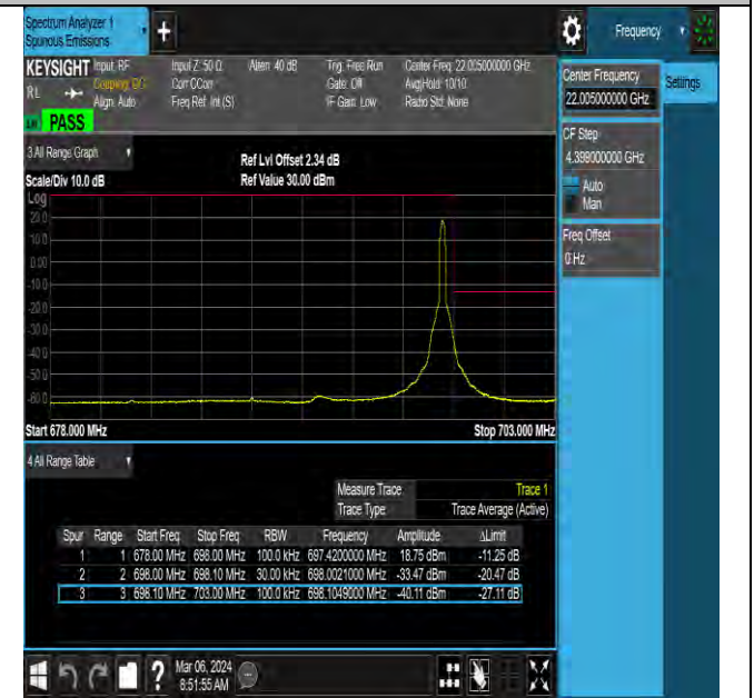
NTNV-N71-PC3-15-20-H-DFT-QPSK-Edge_1RB_Right-Ant0 -PASS
