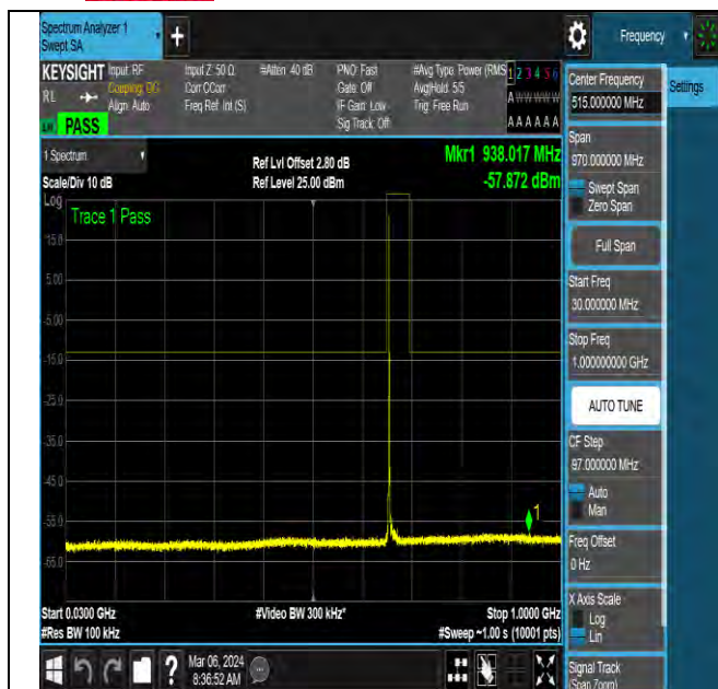
NTNV-N71-PC3-15-20-L-DFT-QPSK-Edge_1RB_Left-Ant0-P ASS
