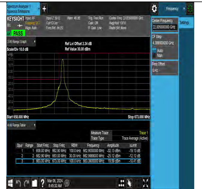
NTNV-N71-PC3-15-10-L-DFT-QPSK-Edge_1RB_Left-Ant0-P ASS
