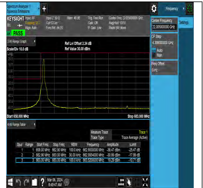
NTNV-N71-PC3-15-20-L-DFT-QPSK-Edge_1RB_Left-Ant0-P ASS
