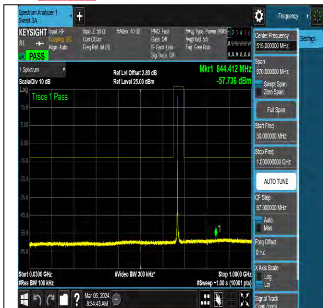
NTNV-N71-PC3-15-10-M-DFT-QPSK-Edge_1RB_Left-Ant0-PASS
