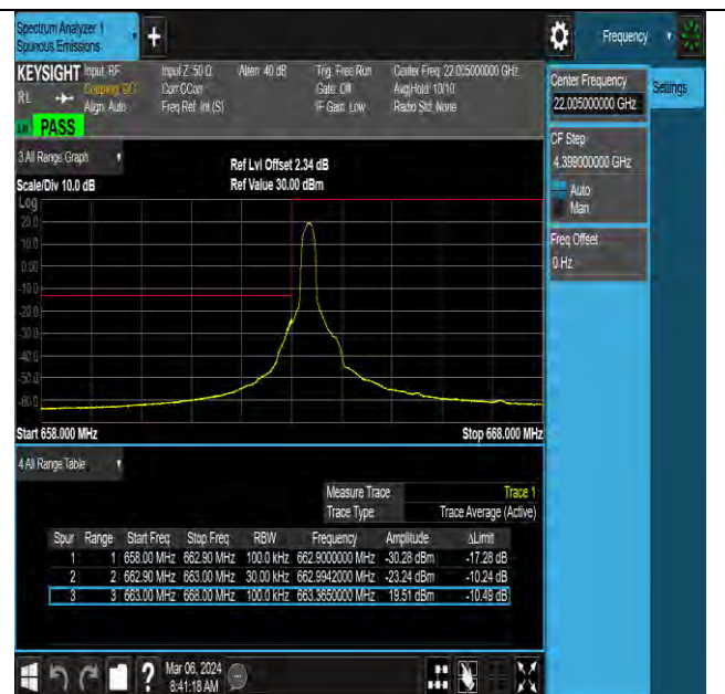
NTNV-N71-PC3-15-5-L-DFT-QPSK-Edge_1RB_Left-Ant0-PASS
