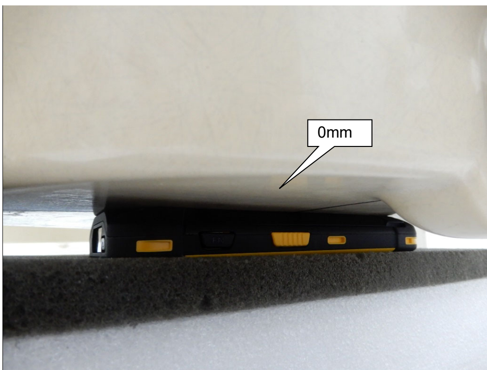
EUT Back_0mm
