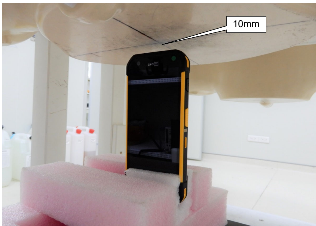
EUT Top_10mm
