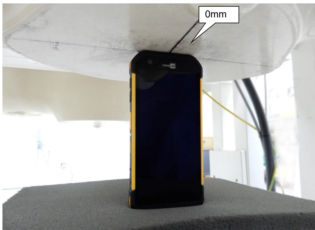
EUT Top_0mm
