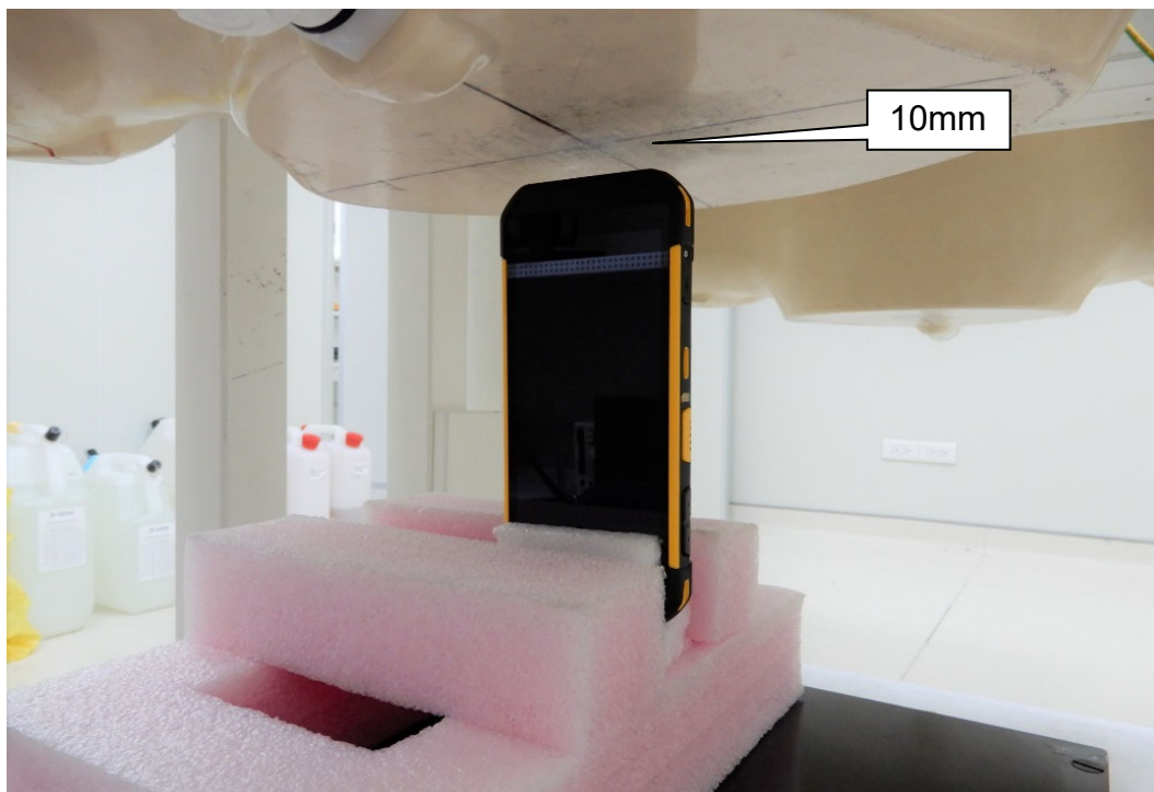
EUT Bottom_10mm
