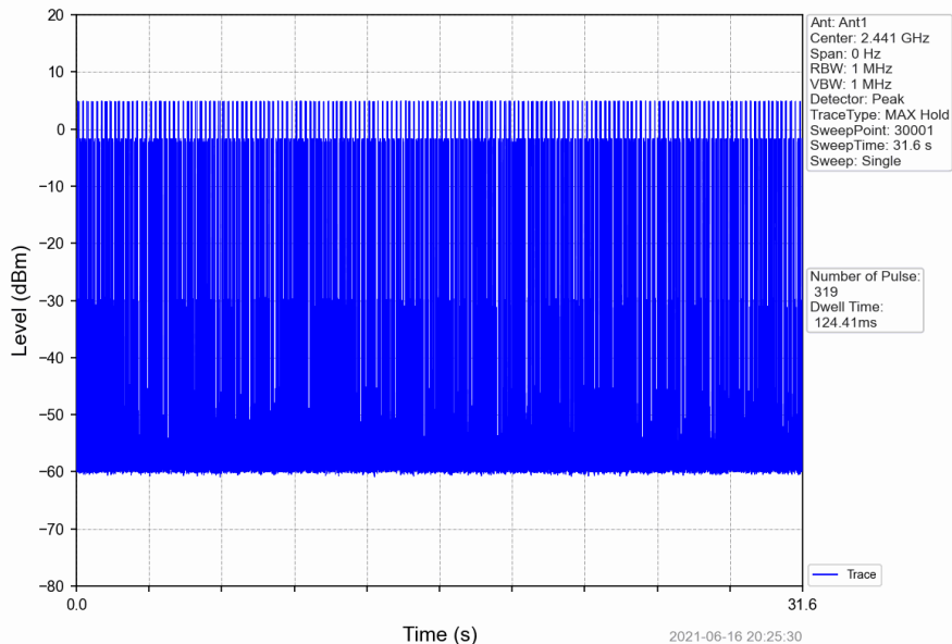
Pi/4DQPSK_2DH1_HOPP_Ant1_NTNV
