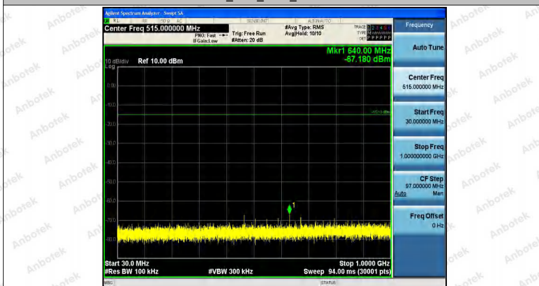
11B_Ant2_2412_30~1000
