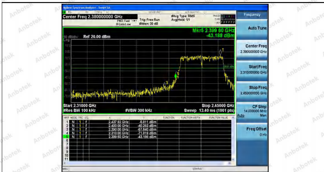
11N40_Ant2_Low_2422
