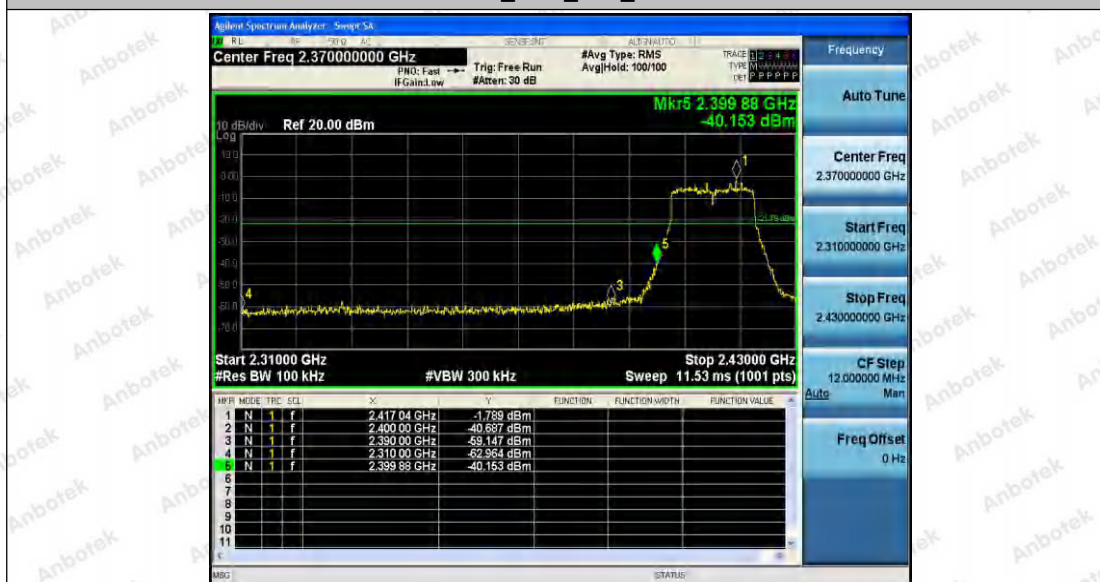
11N20_Ant2_Low_2412
