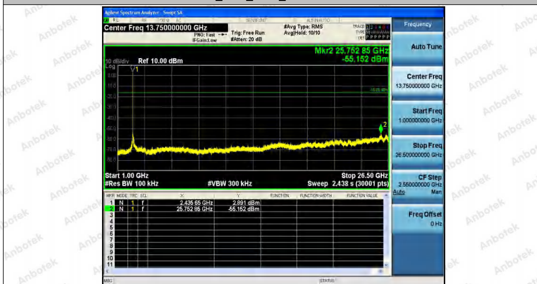
11B_Ant2_2437_0~Reference
