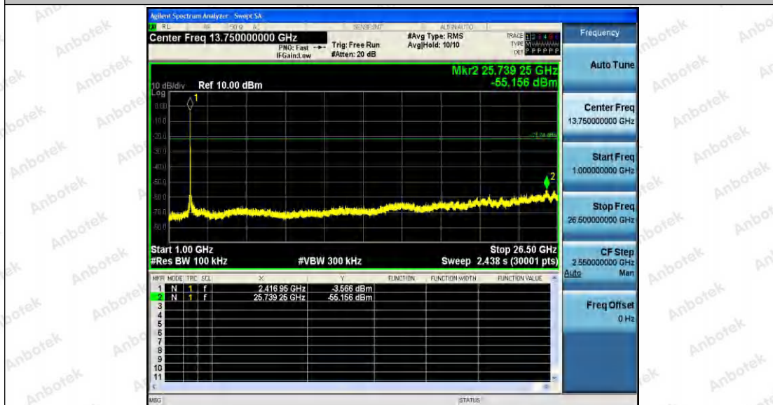
11N20_Ant2_2412_0~Reference
